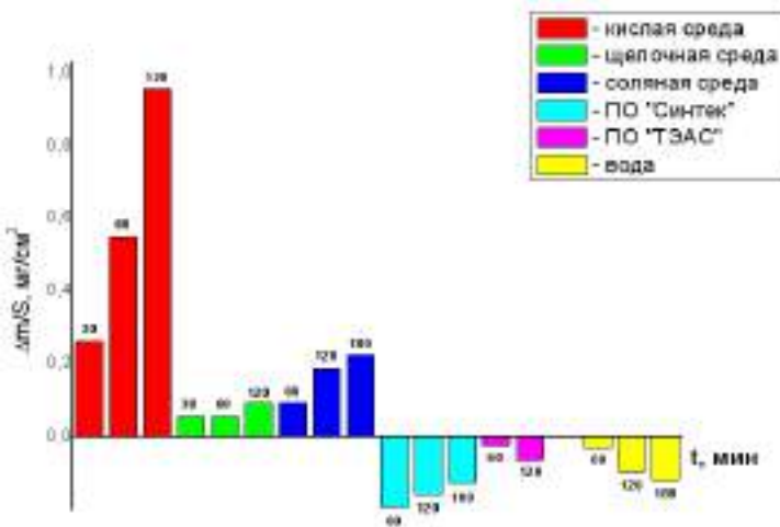
Рисунок 1 – Результаты образования продуктов коррозии на Ст.3 в различных средах
