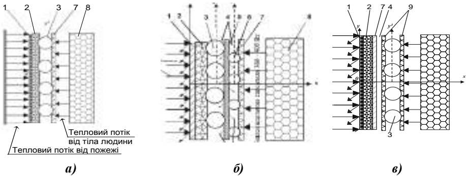
Рис. 2. Конструкції оболонки костюма з однорядним розташуванням трубок (а), із дворядним розташуванням трубок (б) з однорядним розташуванням трубок і повітряним прошарком (в):
