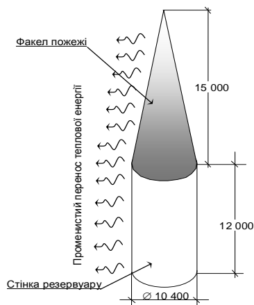
Рис. 3. Схема розташування факелу над резервуаром, що горить
