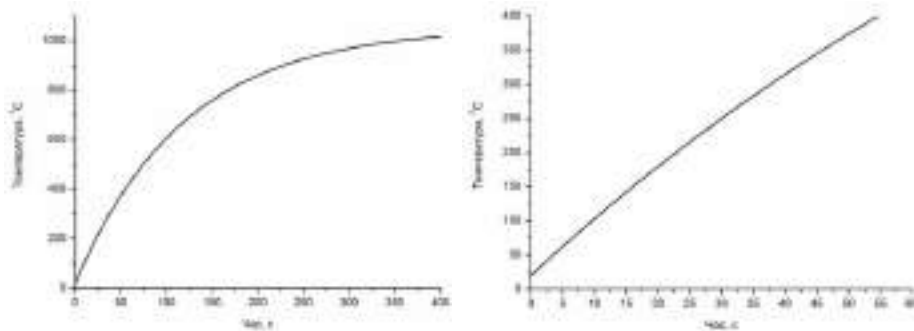
Рис. 1. Зміна температури нагрівання провідника площею поперечного перерізу 1,5 \text{ мм}^2 з часом при струмі КЗ
