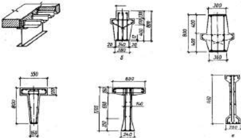
Рис. 1. Поперечні перерізи сталобетонних балок із зовнішнім армуванням: а) сталобетонні плити армовані профільованим сталевим листом; б), в) попередньо напружені ригелі з одним та подвійним полосовим армуванням 1-12,0 м; г), д) попередньо напружені підкранові балки прольотом 6,0, 12,0 м; е) попередньо напружена балка покриття прольотом 12,0 м.
