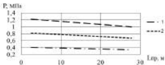
Рис. 2. Залежність необхідного тиску на ПКК від довжини розмотаної з котушки частини рукава та витрати на пожежогашіння: 1 – Q=1,5 л/с; 2 – Q=2,13 л/с; 3 – Q=2,6 л/с.
