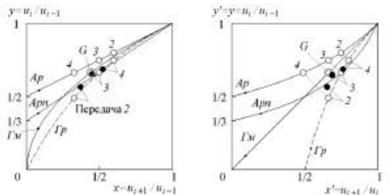
Рисунок 3 — Координатні системи для відображення і аналізу структури рядів передатних відношень
