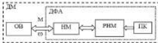
Рис. 1. Функціональна схема стенда для проведення випробувань:
