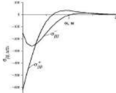
Рисунок 3 – Зміна кільцевих напружень вздовж координати \alpha
