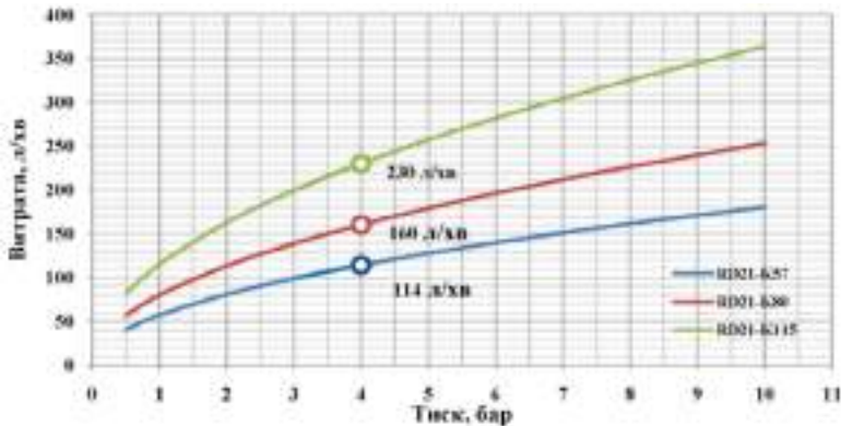
Рисунок 2 – Графік зміни витрати від тиску у дренчерних розпилювачах типу RD21-Kxx; Вказаний розрахунковий розхід при тиску 4 бар: RD21-K57 (1,9 л/с.); RD2- K80 (2,667л/с.), RD21-K115 (3,83л/с.).
