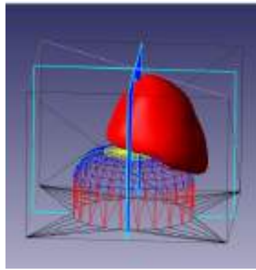
Ізоповерхня 500°C
