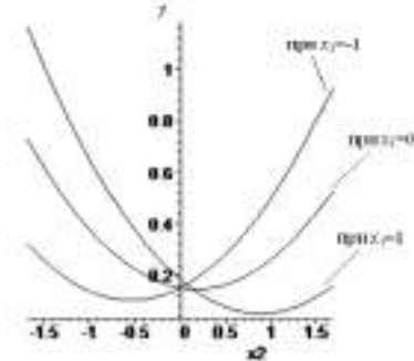
Рис. 1 – Залежність втрат напору в рукаві у від відстані між манометрами x_2 при напорі в мережі x_1 на мінімальному, середньому та максимальному рівнях
