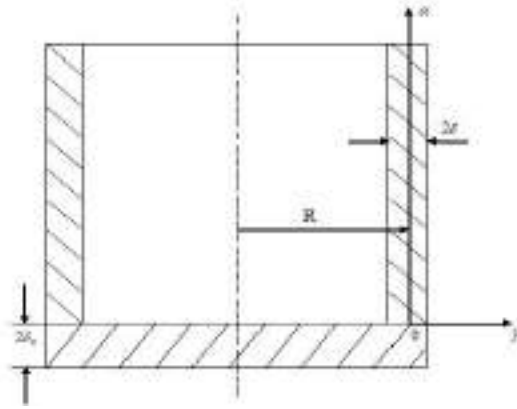
Рис. 1. Осьовий переріз резервуара
