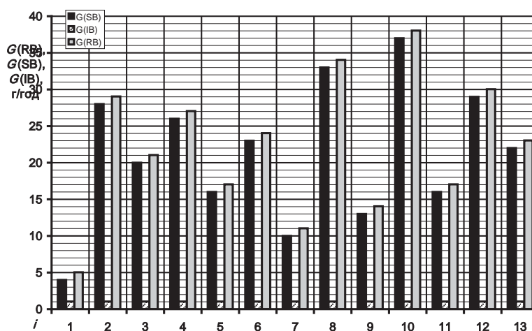
Рис. 2. Розподіл значень масового годинного викиду пари моторного палива при великому і малому диханні резервуара по режимах випробувального циклу ESC для автотракторного дизеля 2Ч110,5/12
