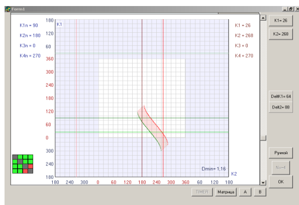
Рис. 4. Выбор безопасного курса K2 второго судна
