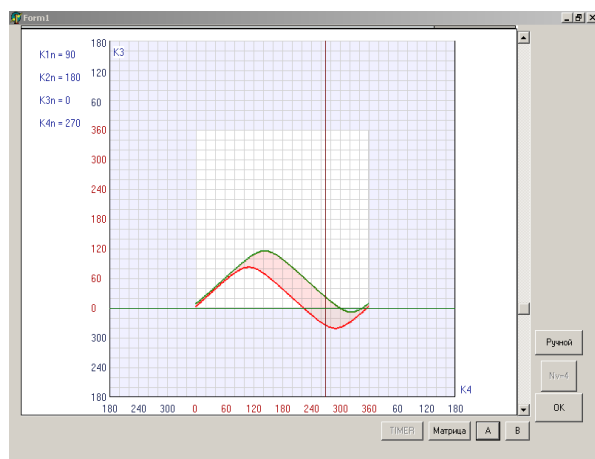
Рис. 5. Область опасных курсов третьего и четвертого судов
