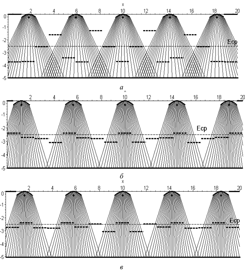
Рис. 2 – Варіанти рівномірного обігріву теплоприймача: a - c = 1,3 м; d = 2,8 м; k = 0,24 ; K_p = 44,6 ; b - c = 1,4 м; d = 3 м; k = 0,3 ; K_p = 15,1 ; в - c = 1,4 м; d = 2,8 м; k = 0,3 ; K_p = 11,3 .
