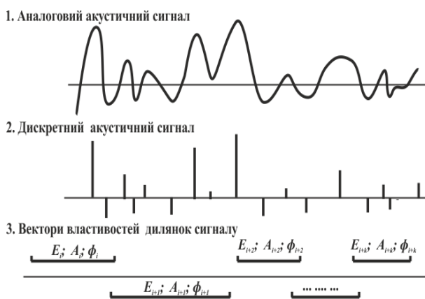
Рис.1. Узагальнена схема обробки акустичного образу з джерела НС унаслідок пожежі на ПНО
