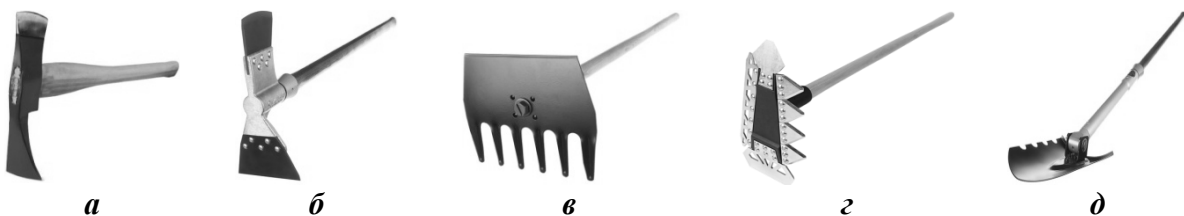
Рисунок 2 – Ручні засоби: а) топор pulaski; б) magnum pulaski; в) граблі McLeod; г) інструмент Gorgui ; д) універсальна лісова лопата.
