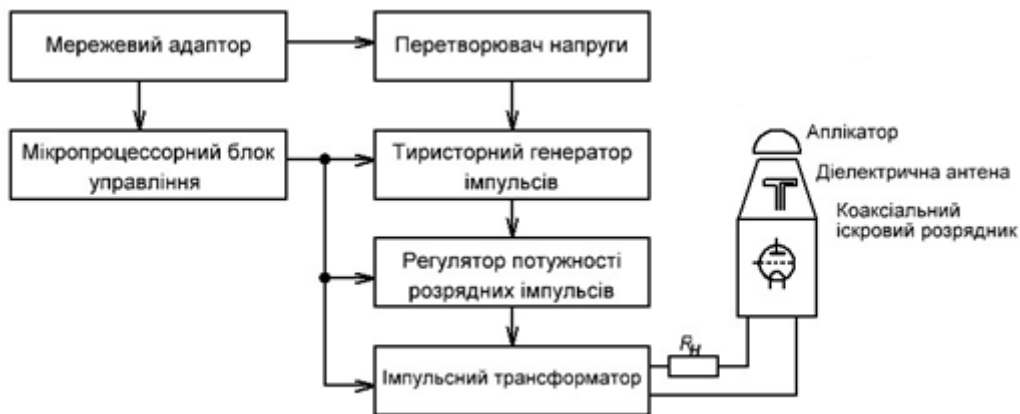
Рис. 2. Макет імпульсного генератора іскрових розрядів
