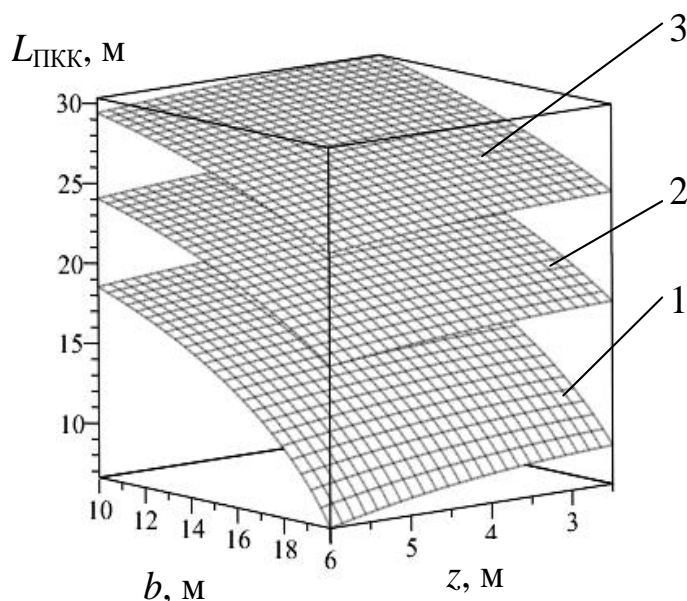
Рис. 2. – Залежність максимально можливої відстані між ПКК ( L ) від ширини ( b ) та висоти ( z ) приміщення (за умовою захисті всієї ширини приміщення) для пожежних рукавів довжиною: 1- 10 м, 2 – 15 м, 3 – 20 м.
