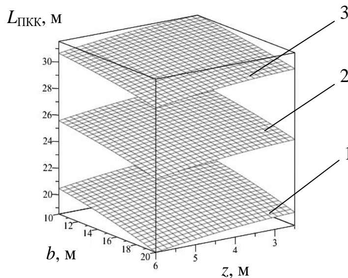
Рис. 1. – Залежність максимально можливої відстані між ПКК ( L_{\text{ПКК}} ) від ширини ( b ) та висоти ( z ) приміщення (за умовою половини ширини приміщення) для пожежних рукавів довжиною: 1- 10 м, 2 – 15 м, 3 – 20 м.
