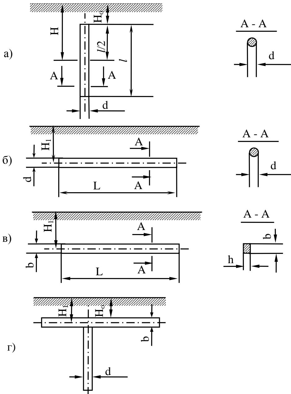
Рис. 2.1 – Елементи штучного заземлювача:
