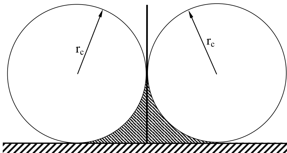
Рис. 2.2 – Переріз у вертикальній площині об'єму, який захищається вертикальним стрижневим перехоплювачем (розраховано методом сфери, що котиться)
