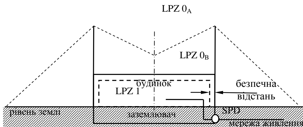
Рис. 3.4 – Зони захисту від вторинних дій блискавки при застосуванні для захисту від прямих влучень блискавки розрахованої системи перехоплення
