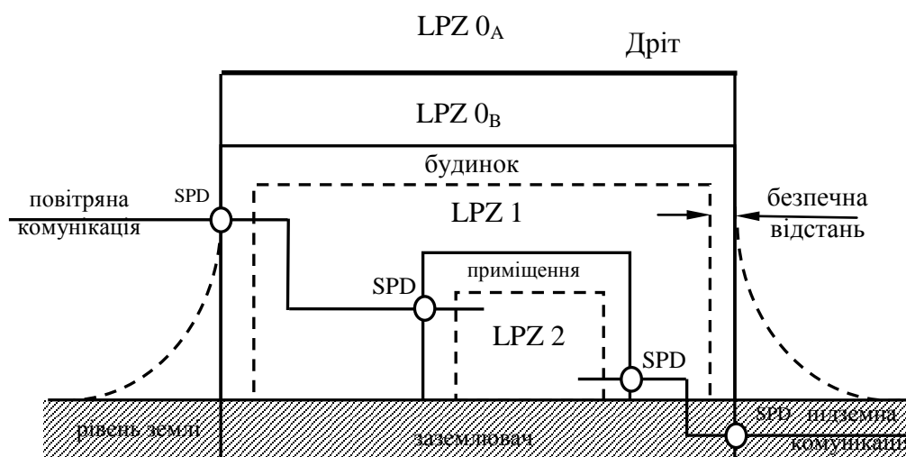
Рис. 2.7 – Зони захисту від вторинних дій блискавки при застосуванні для захисту від прямих влучень блискавки дротової системи перехоплення
