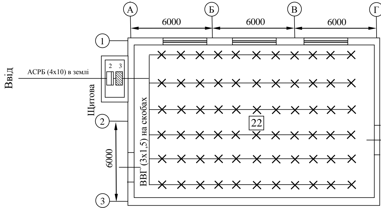
Специфікація освітлювального обладнання
