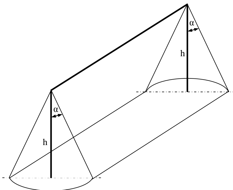
Рис. 2.4 – Об’єм, що захищається вертикальним стрижневим перехоплювачем (розрахований методом захисного кута)
