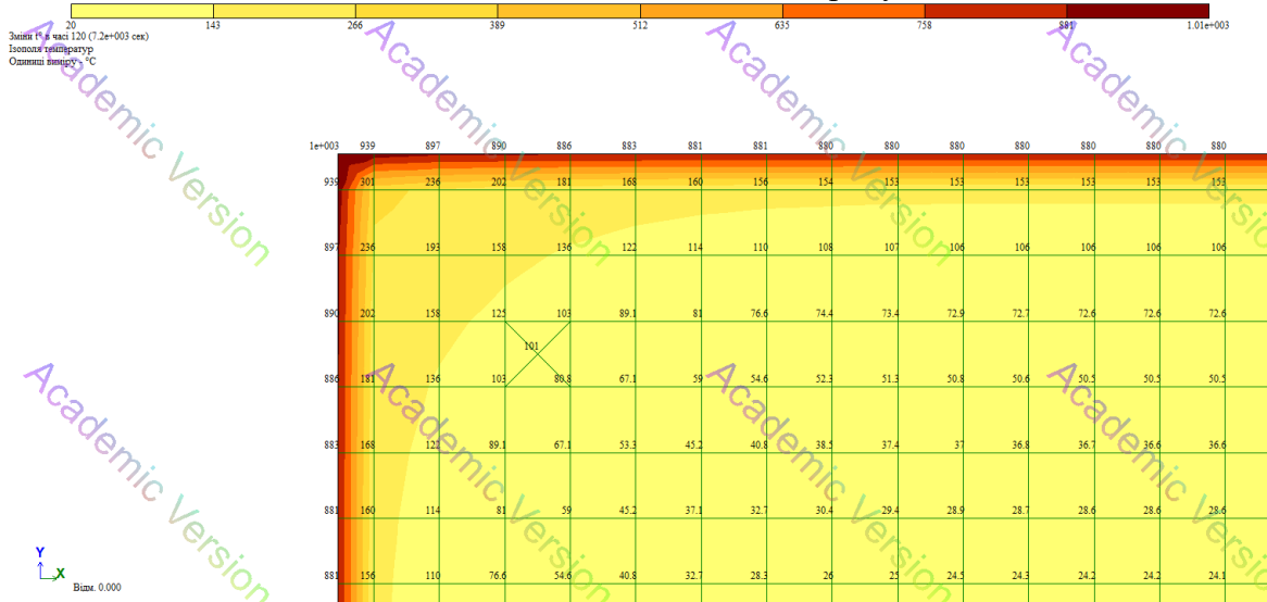
Рис. 2. Розподіл температур у вогнезахисненій залізобетонній колоні на 120 хвилині випробування
