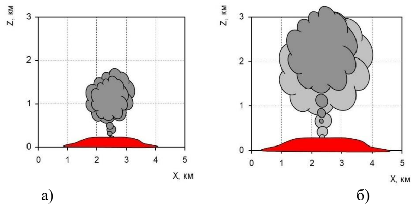
Рис. Приклад розрахунків утворення та випадіння радіоактивних продуктів згоряння під час лісових пожеж у містах Прип'ять (а) та Чорнобиль (б)
