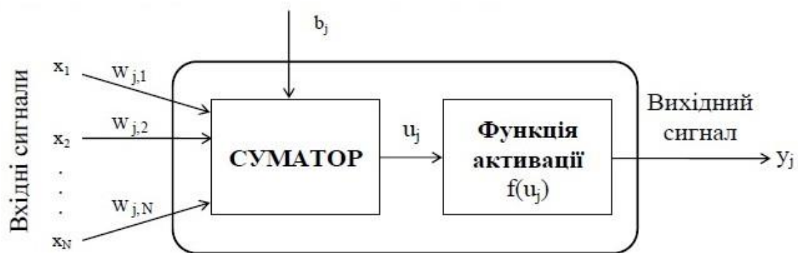
Рис. 1. Схема штучного нейрона
