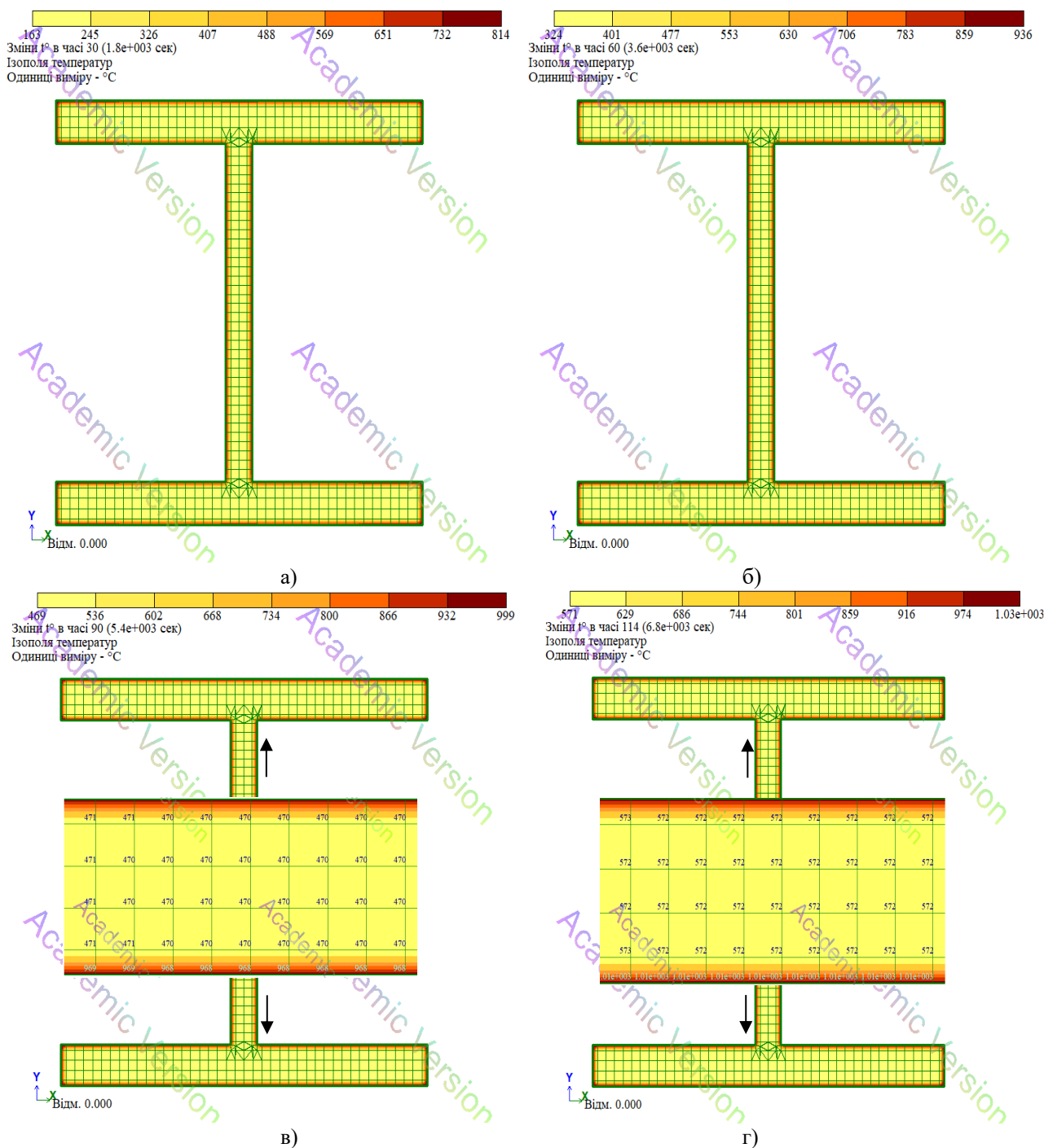
Рисунок 7 – Розподіл температур в вогнезахисній сталевій колоні на 30 (а), 60 (б), 90 (в) та 114 (г) хвилині випробування
