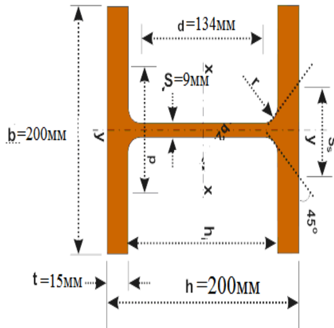
Рисунок 6 – Геометричні розміри сталевій колони для моделювання
