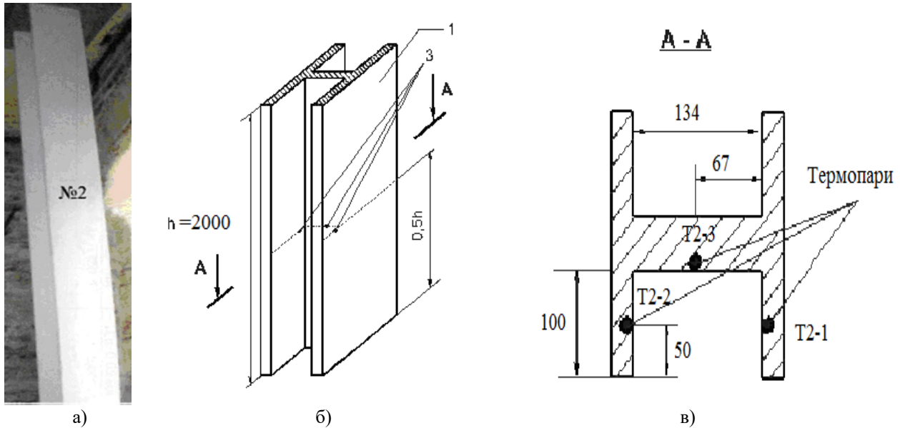
Рисунок 1 – Загальний вигляд вогнезахисної колони (а) та схема розташування термометрів на колоні (б, в), які випробовуються без навантаження
