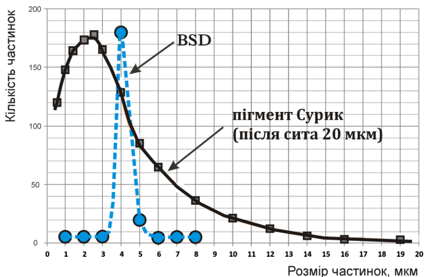
Рис. 1 – Гістограма розподілу частинок за розмірами для типового пігменту «Сурик» та нетрадиційного наповнювача BSD
