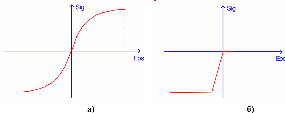
Рис. 4. Закони нелінійного деформування бетону: а – експонентний; б – кусково-лінійний
