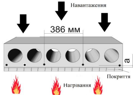
Рис. 1. Схема температурних та статичних навантажень на плиту
