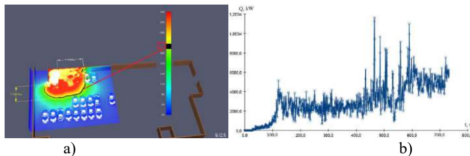
Рис. 2. Моделювання пожежі електромобіля та зарядної станції: а – фрагмент розвитку пожежі та теплові розподіли на суміжному до машинісця із зарядною станцією для електромобілів об'єкті на 610 с пожежі, б – відтворений режим швидкості виділення тепла під час дослідження процесів горіння електромобіля обладнаного літій-іонними акумуляторами та зарядної станції.
