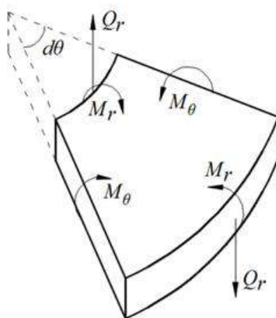
Рис. 1. Зусилля в кільцевій пластині.
