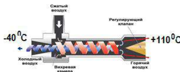
Рис. 1. Трубка Ранка-Хілша.
