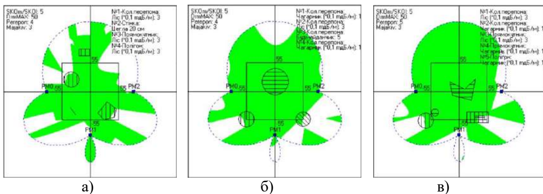
Рис. 2. Робоча зона RTLS-системи при наявності: а) 4 перепонов перетину типу «коло», «стінка», «прямокутник» та «багатокутник»; б) 3 колових перепонов з різних матеріалів; в) перепонові складної форми.
