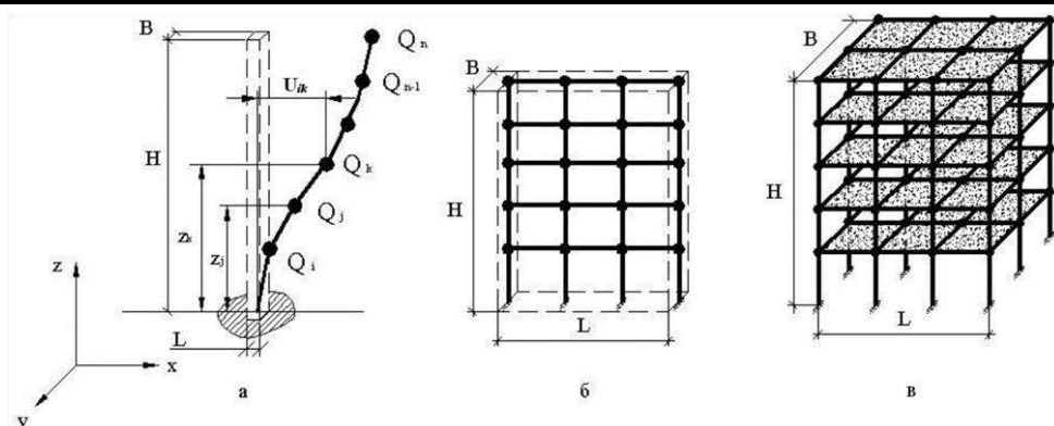
Рис. 1. Розрахункова схема у вигляді пружно-деформованих стержнів.
