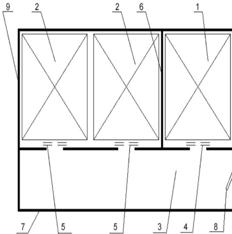
Рис. 6.4. – Приклад розташування пожежного ліфта у відокремленій шахті із загальним ліфтовим холлом з іншими ліфтами
