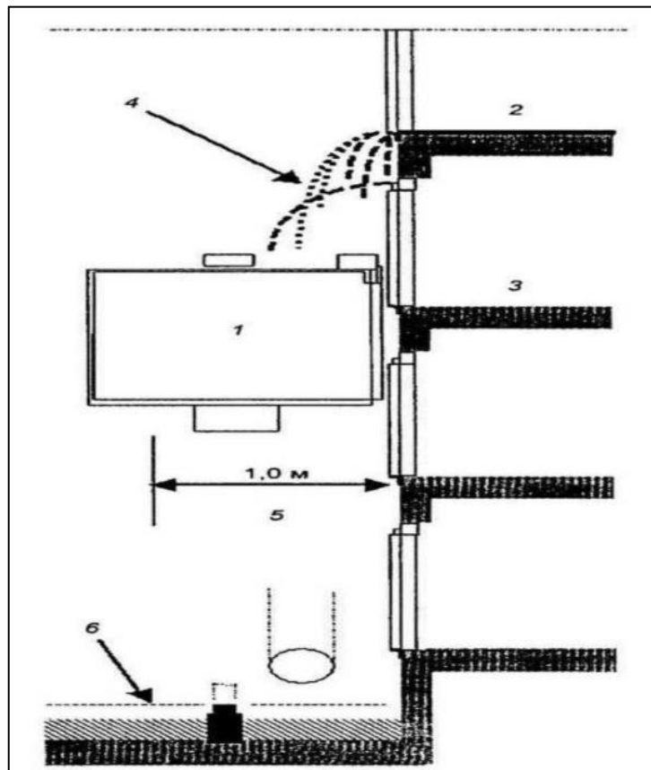
Рис. 6.2 – Захист електроустаткування від вогнегасної речовини
