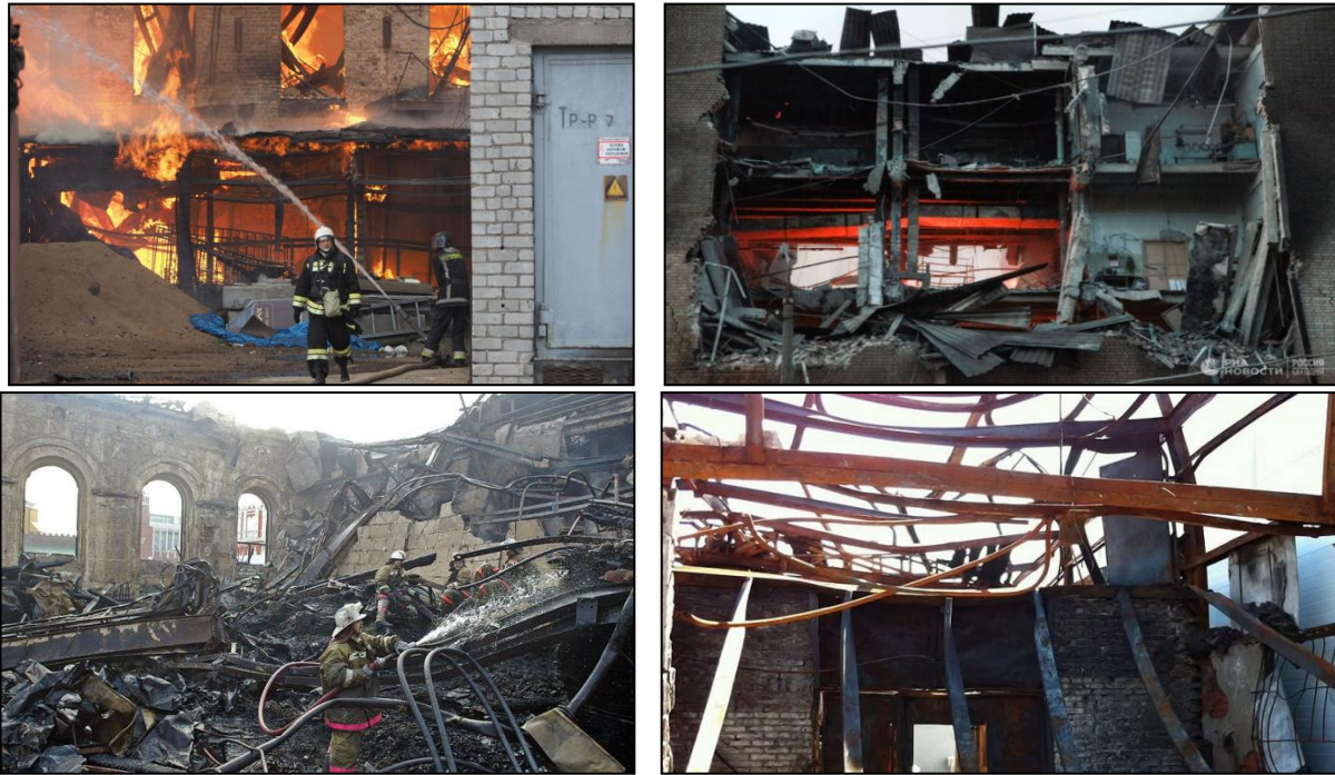
Рис. 7.1 – Наслідки руйнування будівель через втрату несучої здатності будівельних конструкцій під дією високих температур
