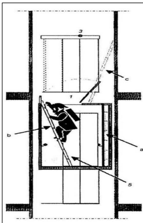
Рис. 6.9 - Самостійне рятування з використанням пересувної драбини, яку зберігають у шафі кабіни
