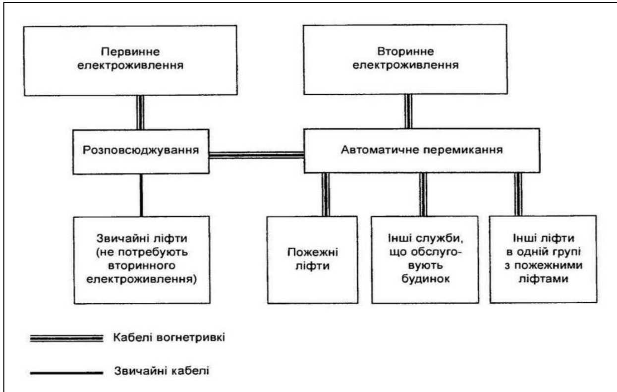
Рис. 6.7 - Типи електроживлення пожежних ліфтів
