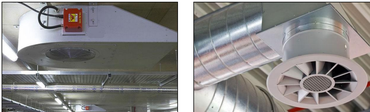
Рис. 3.6 – Елементи системи димовидалення
