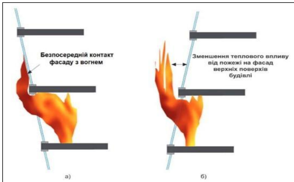
Рис. 9.3 - Приклади теплового впливу пожежі на фасад будівлі за кута ухилу площини фасаду відносно горизонталі (або площини перекриття будівлі):
