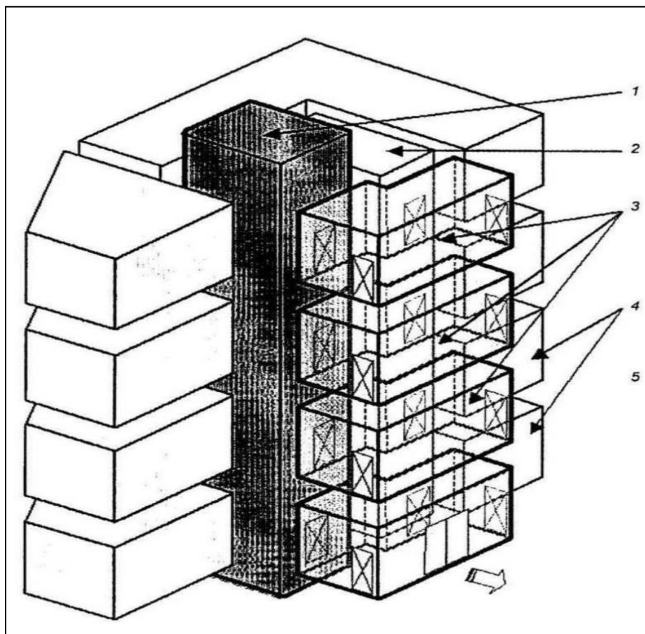
Рис. 6.5 - Принцип протипожежних відсіків
