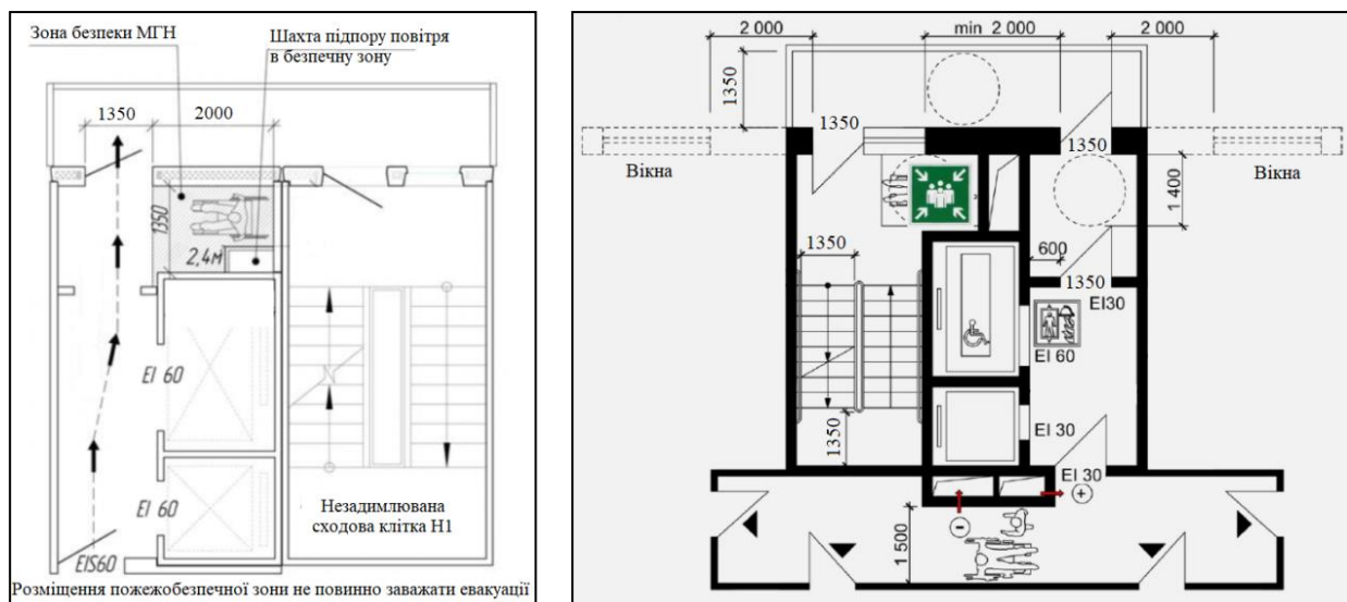
Рис. 5.3 – Приклад виконання пожежобезпечних зон
