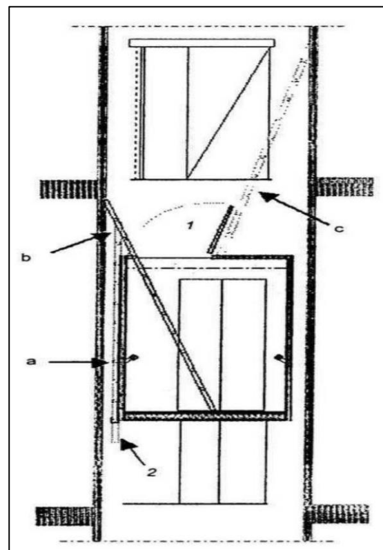
Рис. 6.7 - Рятування ззовні за допомогою драбини, розташованої на кабіні ліфта
