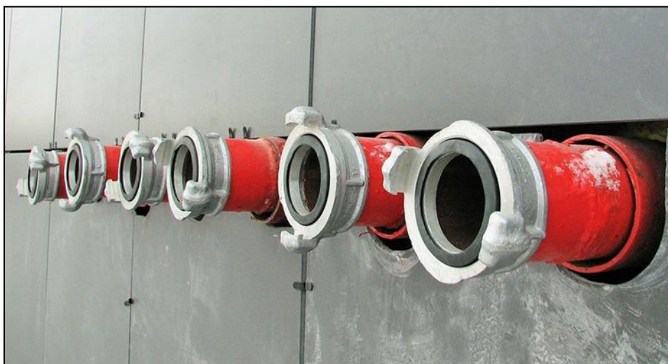
Рис. 9.5 – Пожежні патрубки для приєднання рукавів та подачі води від пересувної протипожежної техніки
