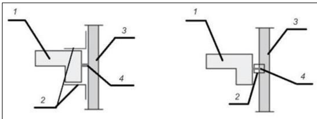
Рис. 9.2 – Приклад улаштування захисних конструкцій фасаду
