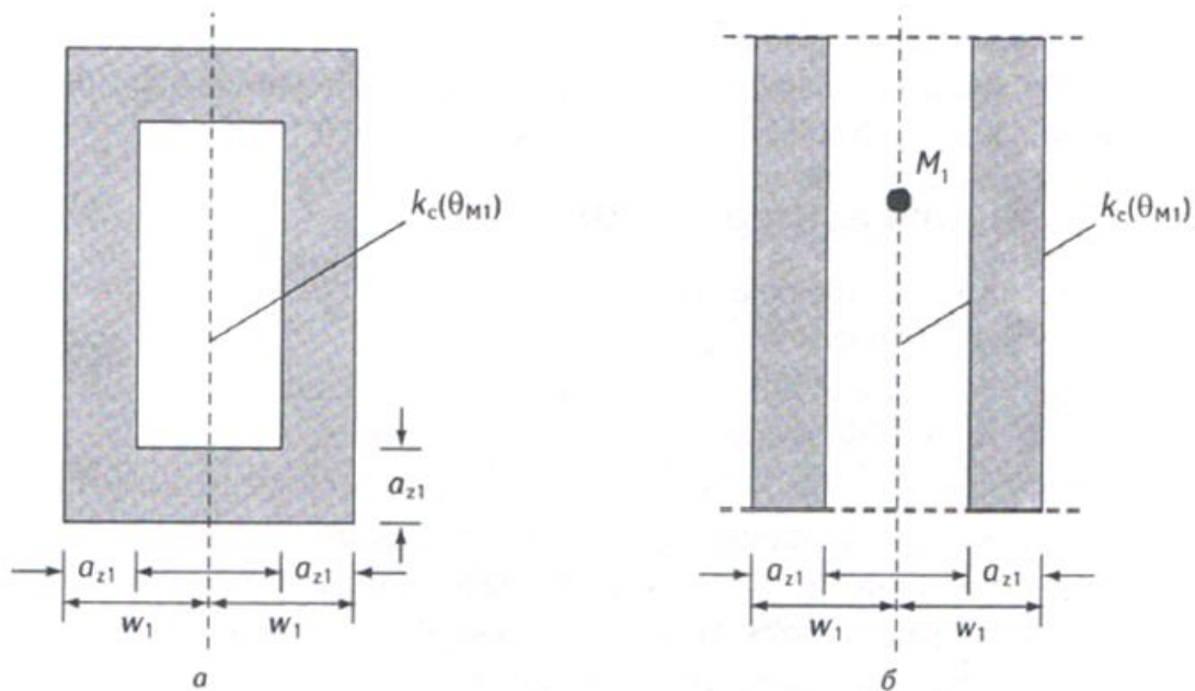
Рисунок 13.6 - Визначення зменшеного поперечного перерізу бетону для залізобетонних колон:
