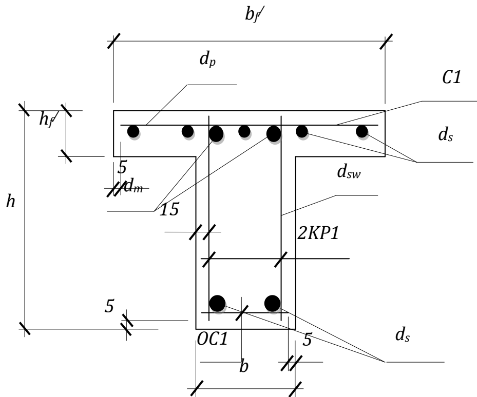
Рисунок 12.2 – Армуння балки таврового перерізу
