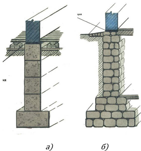
Рисунок 2.8 – Стрічковий фундамент зі збірних блоків (а) та фундамент з бутової кладки (б)
