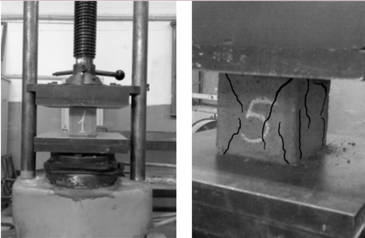
Рисунок 7.1 – Випробування куба для визначення класу бетону
