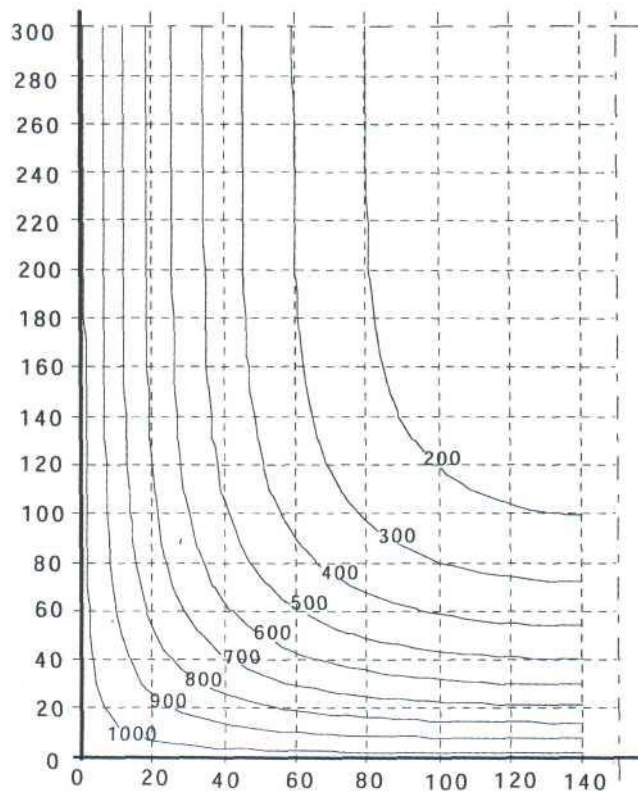
Рисунок 6.11 – Температурні криві балки h \times b = 600 \text{ мм} \times 300 \text{ мм} – R 120, °C
