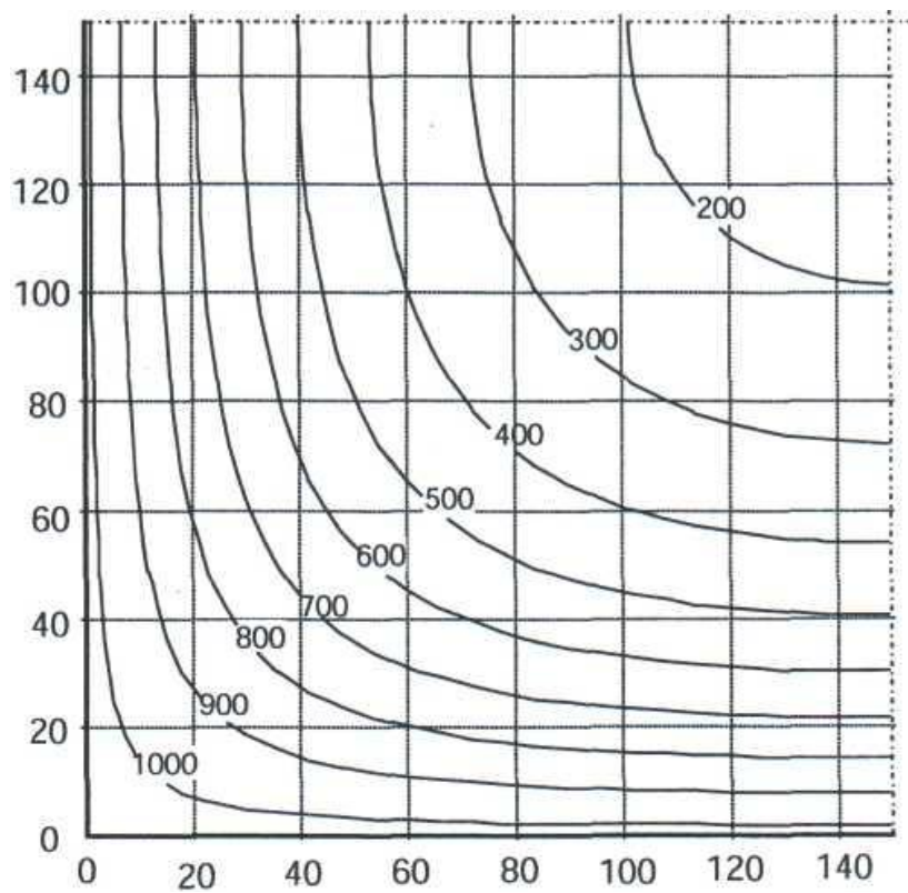
Рисунок 6.17 – Температурні криві колони h \times b = 300 \text{ мм} \times 300 \text{ мм} – R120, °C
