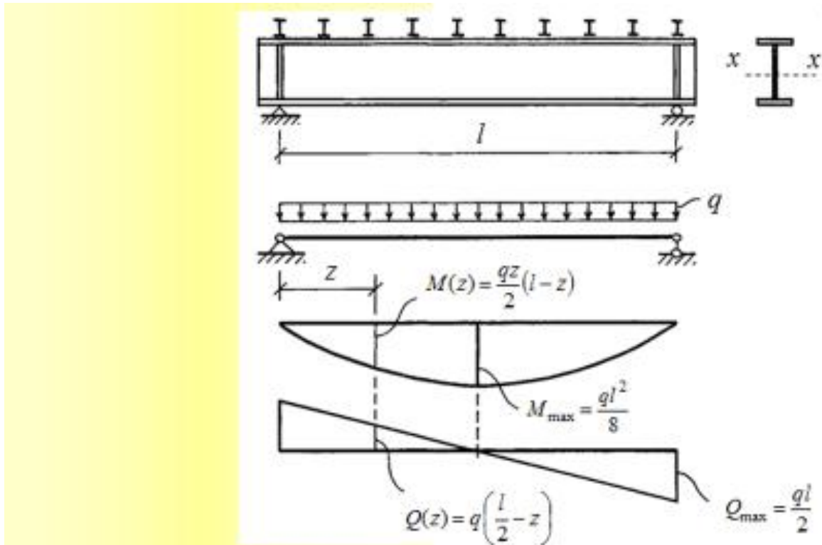
Рисунок 9.6 – Внутрішні зусилля в балці при плоскому згині
