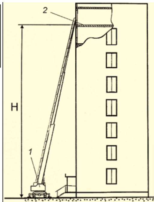
Рисунок 1.20 – Умовна висота будівлі
