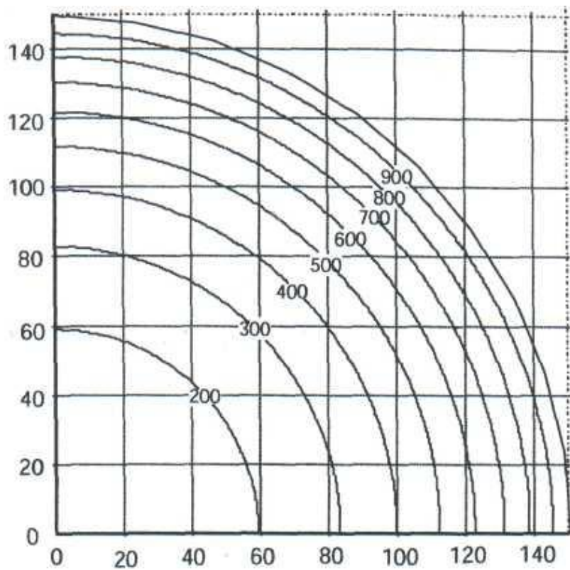
Рисунок 6.21–Температурні криві круглої колони діаметром 300 мм – R90,°C
