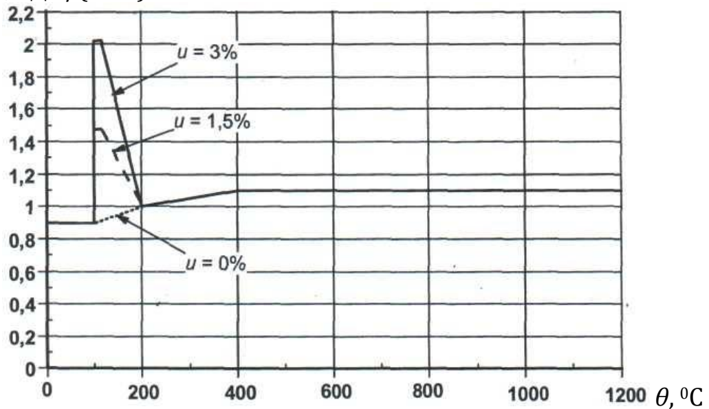
Рисунок 11.4а – Питома теплоємність:
