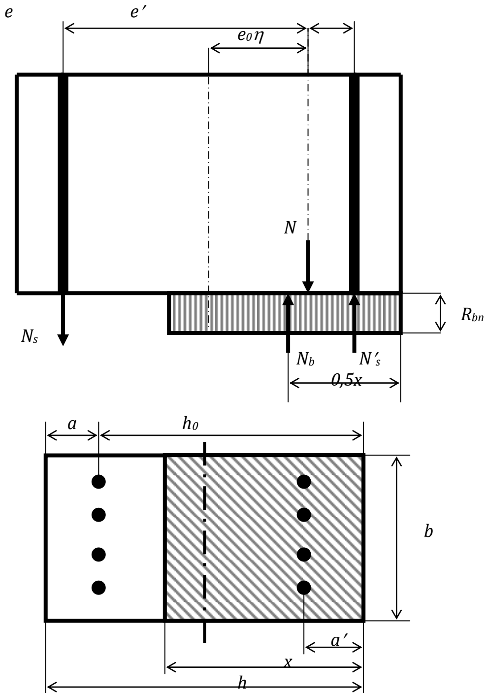
Рисунок 13.4 – Розрахункова схема залізобетонної колони для випадку 2
