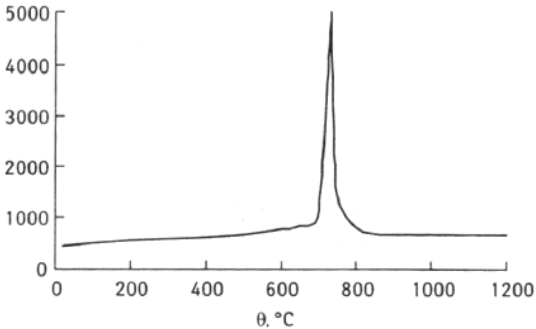
Рисунок 11.9 – Питома теплоємність
