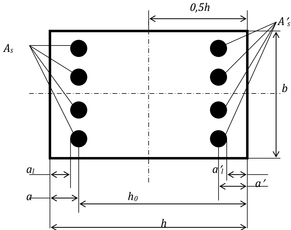
Рисунок 13.2 – Перетин залізобетонної колони
