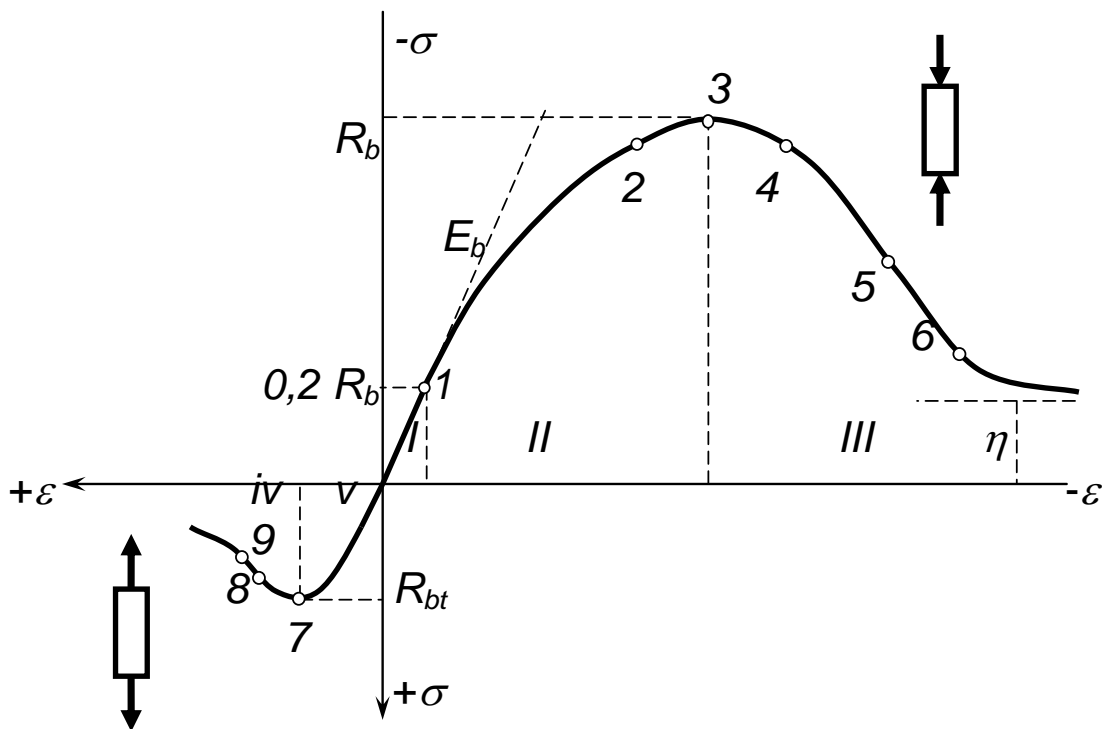
Рисунок 7.3 – Повна діаграма деформування бетону
