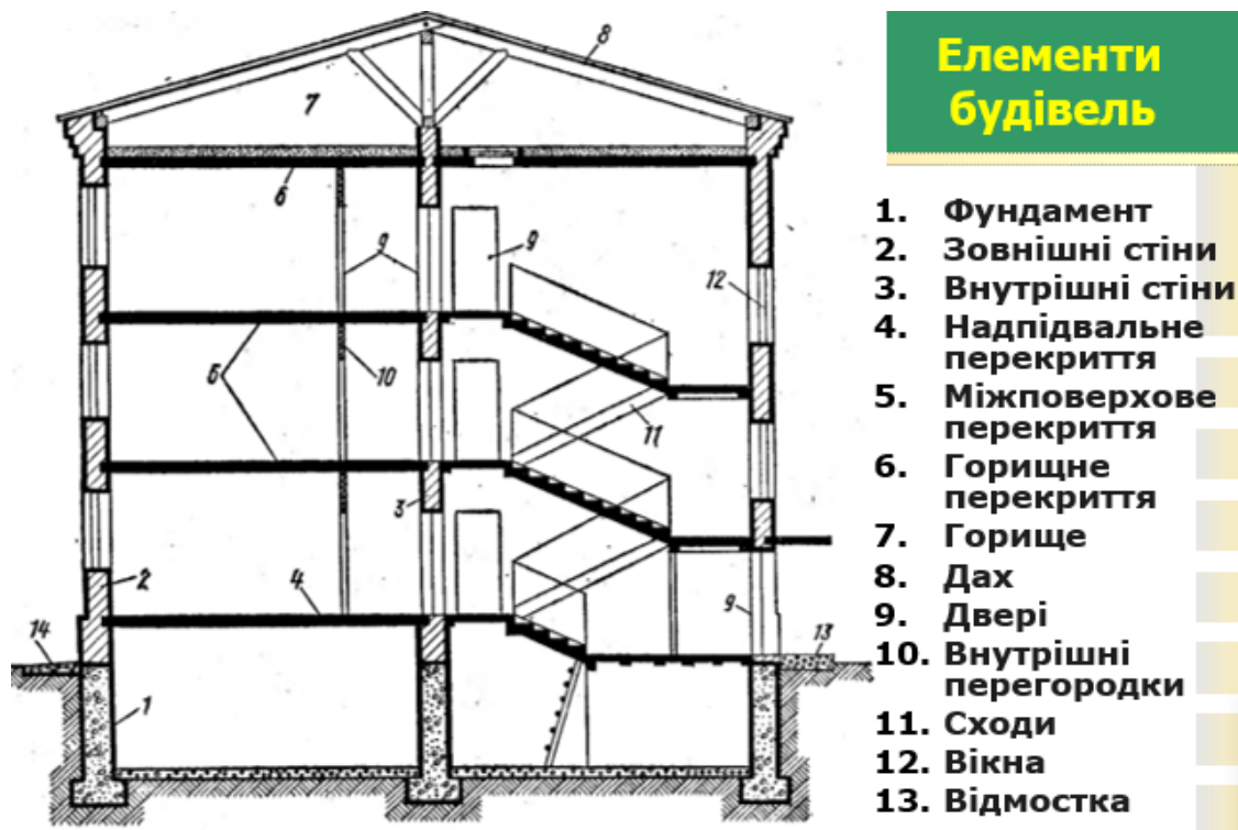
Рисунок 2.3 – Конструктивні елементи будівель
