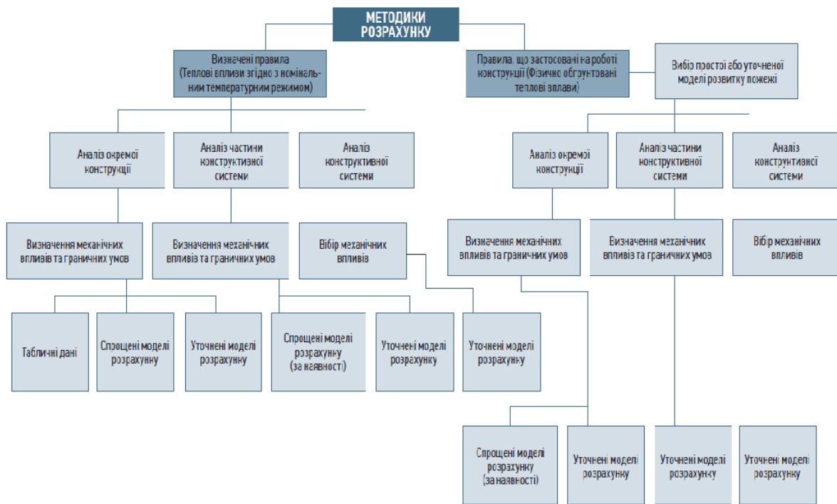
Рисунок 5.1 – Загальний вигляд методики розрахунку на вогнестійкість
