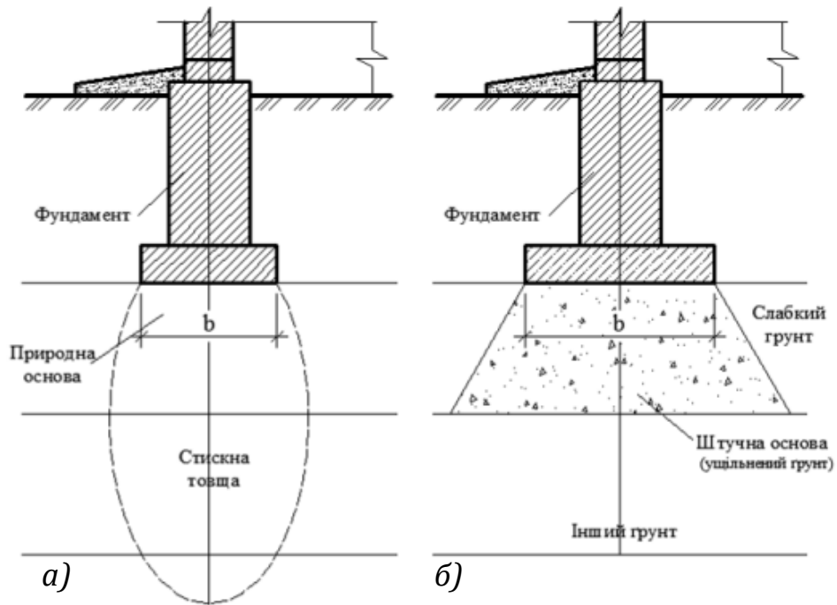
Рисунок 2.5 – Загальний вигляд основ та фундаментів: а – природна основа; б – штучна основа
