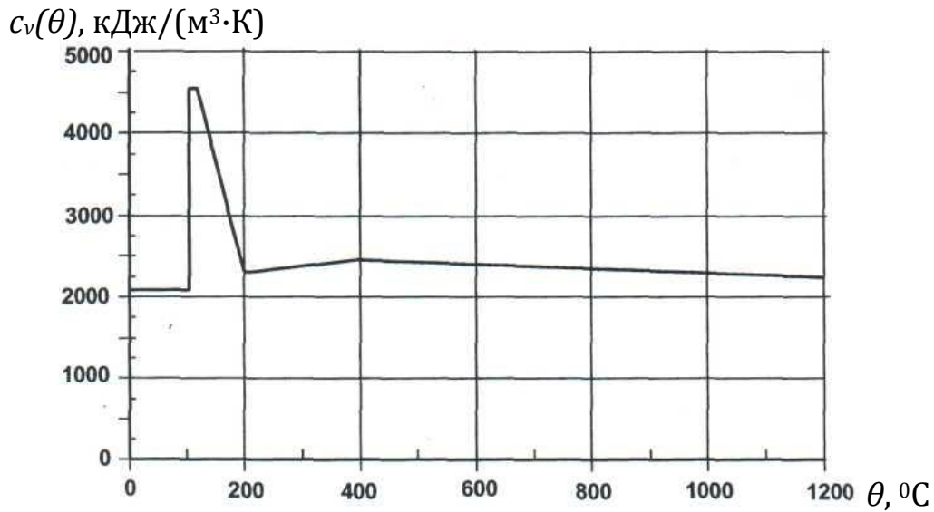
Рисунок 11.46 – Питома теплоємність та об’ємна теплоємність: б) Залежність об’ємної теплоємності c_v(\theta) бетону на силікатному заповнювачі із вологістю u=3\% та густиною більше 2300 \text{ кг/м}^3 від температури
