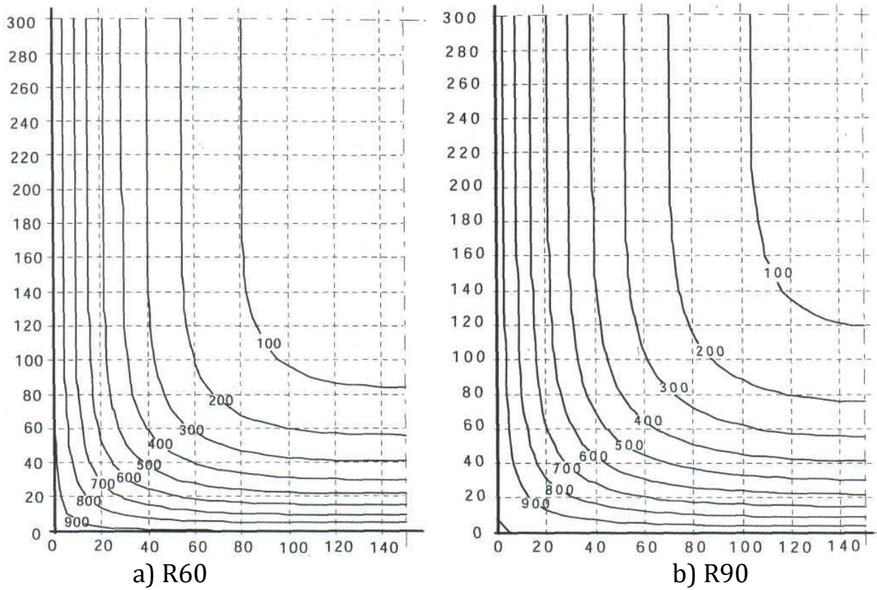
Рисунок 6.10 – Температурні криві балки h \times b = 600 \text{ мм} \times 300 \text{ мм} , °C
