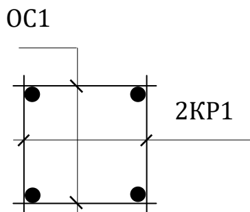
Рисунок 8.7 – Просторовий каркас
