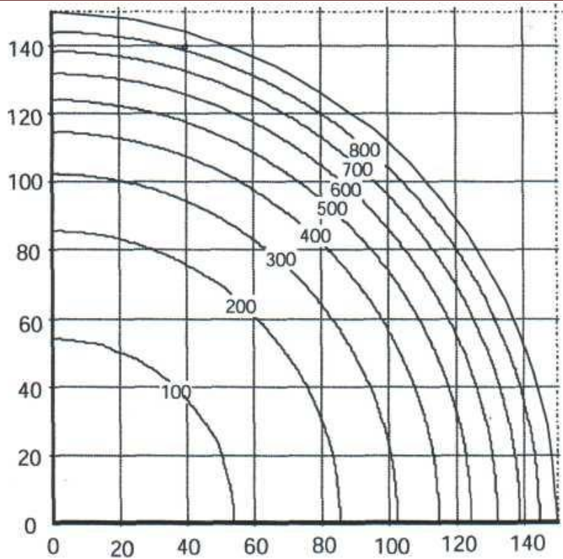
Рисунок 6.20–Температурні криві круглої колони діаметром 300 мм – R60,°C
