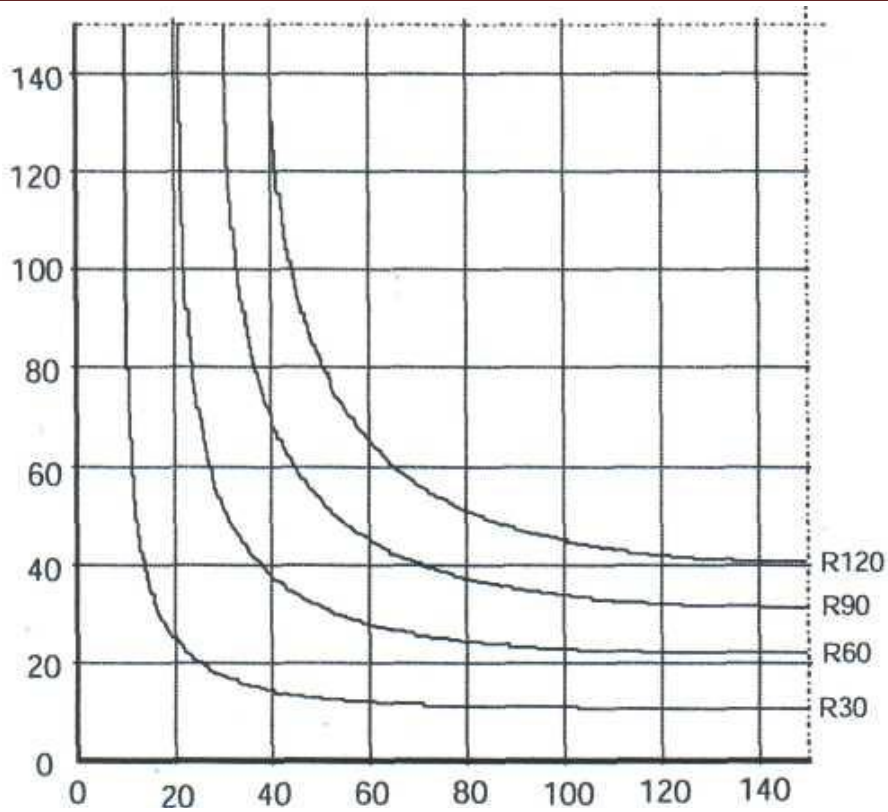
Рисунок 6.18 – Ізотерма 500 °С колони h \times b = 300\text{мм} \times 300\text{мм}
