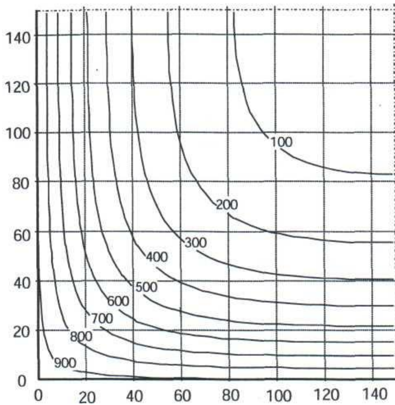
Рисунок 6.15 – Температурні криві колони h \times b = 300 \text{ мм} \times 300 \text{ мм} - R60, ^\circ\text{C}
