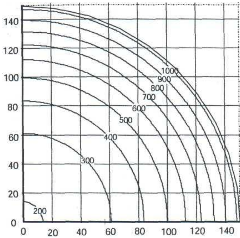
Рисунок 6.22–Температурні криві круглої колони діаметром 300 мм–R120,°C
