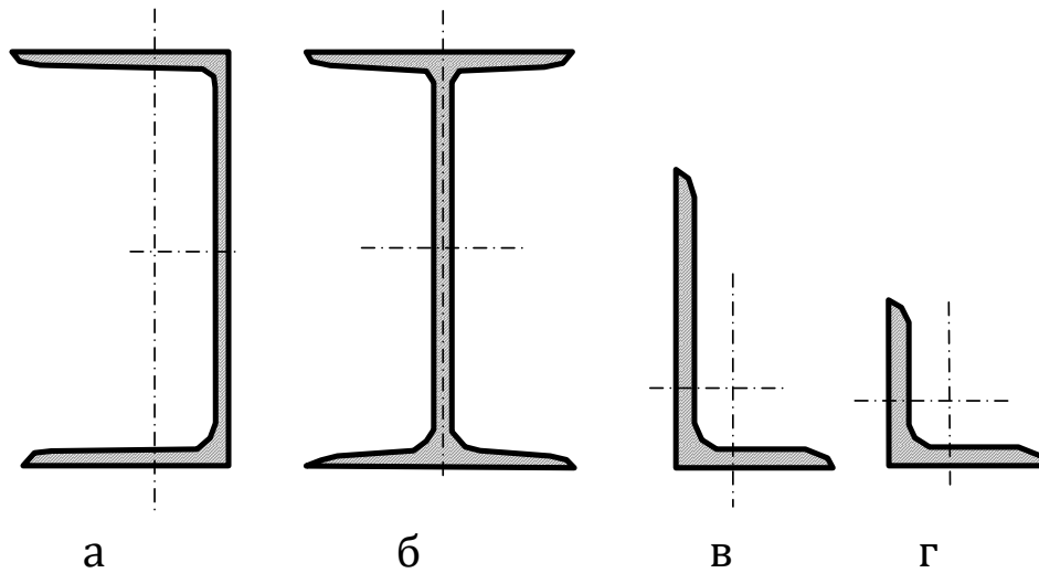
Рисунок 8.1 – Стандартні профiлі сталевого прокату:
