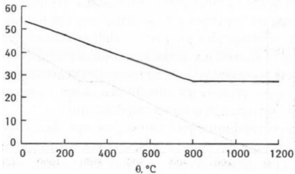
Рисунок 11.10 – Теплопровідність сталі
