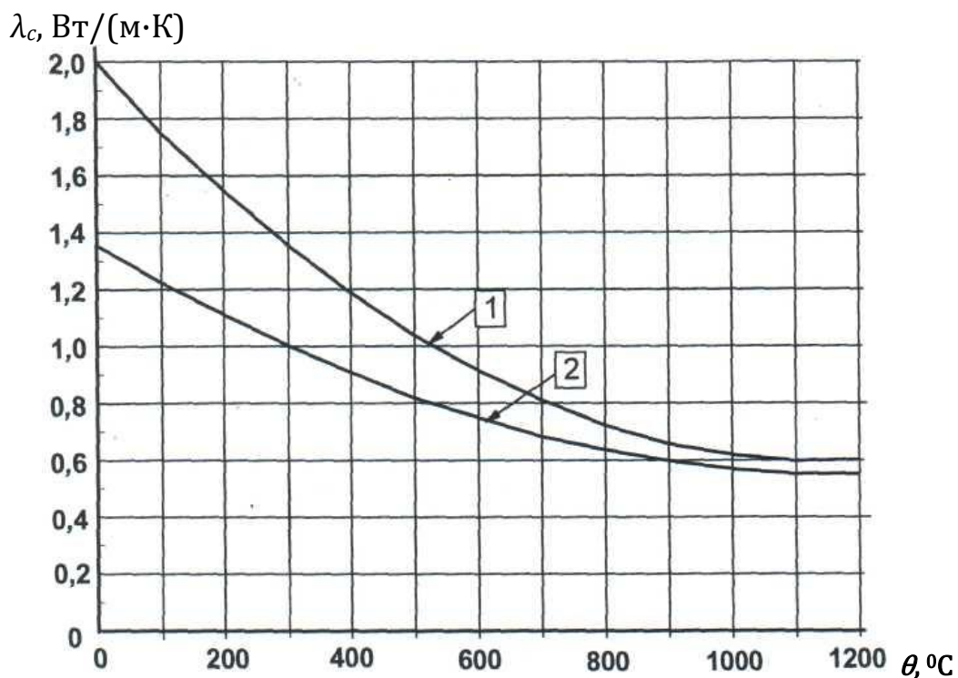
Рисунок 11.5 – Теплопровідність бетону: 1 – верхня межа; 2 – нижня межа
