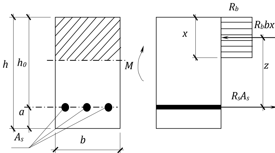
Рисунок 12.3 – Розрахункова схема нормального перерізу при розрахунках міцності прямокутних елементів з одиночним армуванням
