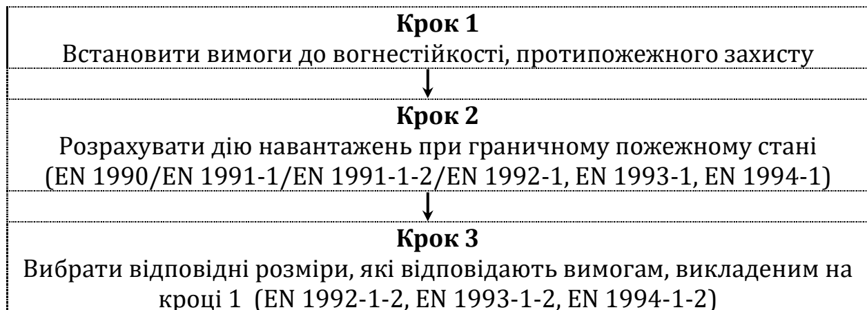
Рисунок 5.2 – Спрощена процедура проектування вогнестійкості конструкцій будівель і споруд
