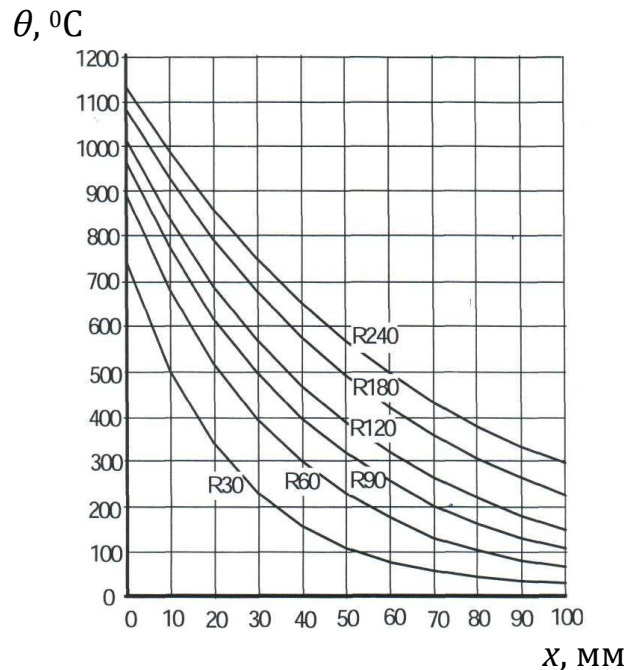
Рисунок 6.5 – Температурні криві плит (висота h=200 мм) для R60 – R240
