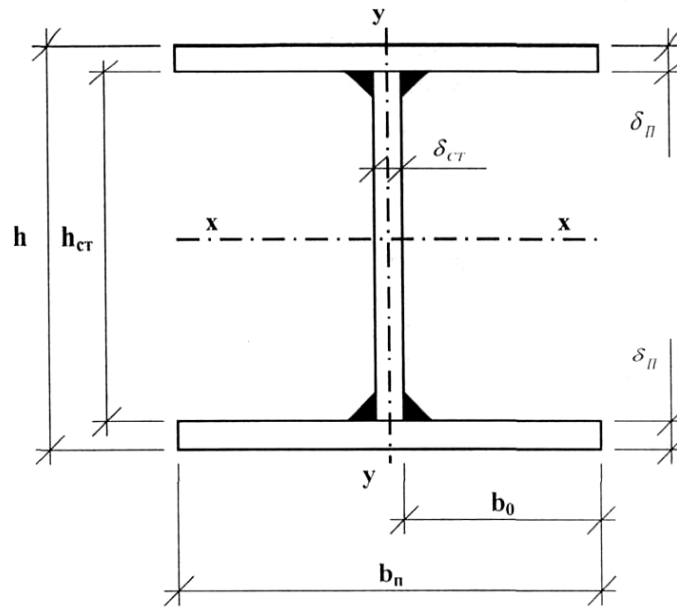
Рисунок 10.2 – Переріз суцільної колони двотаврового профілю:
