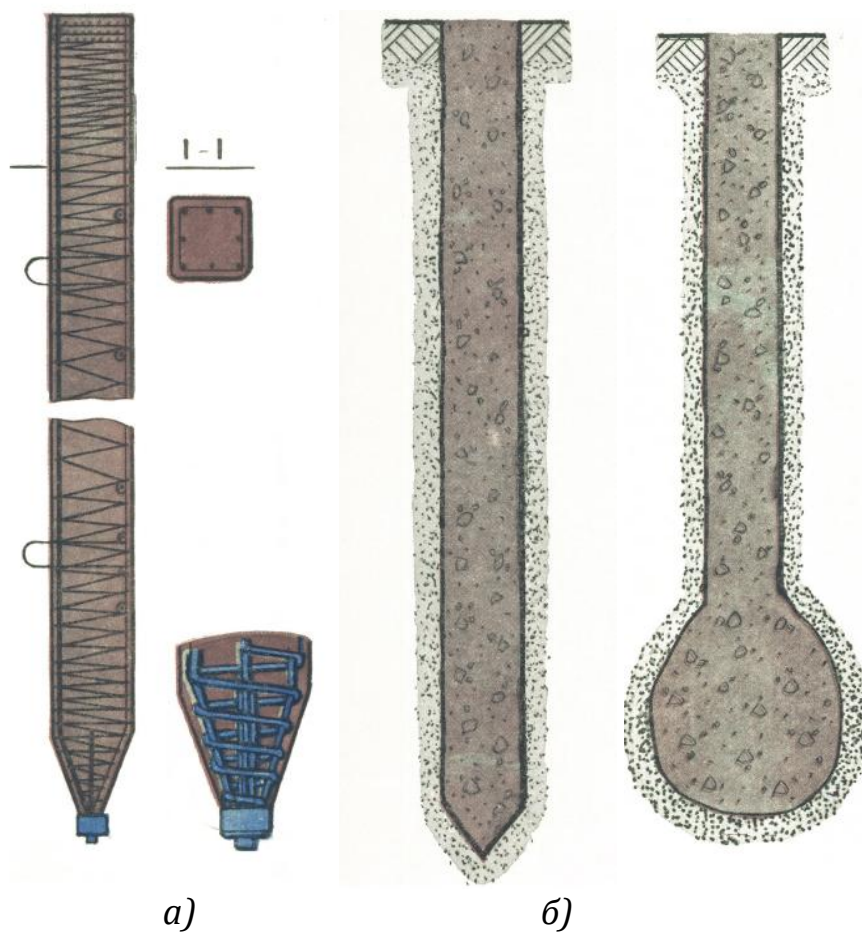
Рисунок 2.6 – Забивні (а) та набивні палі (б)
