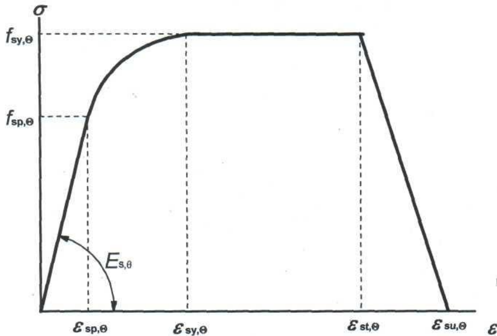
Рисунок 11.7 – Математична модель діаграми «напруження-деформація» для ненапруженої та попередньо напруженої арматури за підвищених температур (позначення для попередньо-напруженої арматури «р» замість «s»)
