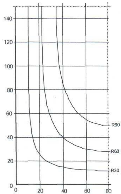
Рисунок 6.9 – Ізотерма 500 °C балки h \times b = 300 \text{ мм} \times 160 \text{ мм} , °C
