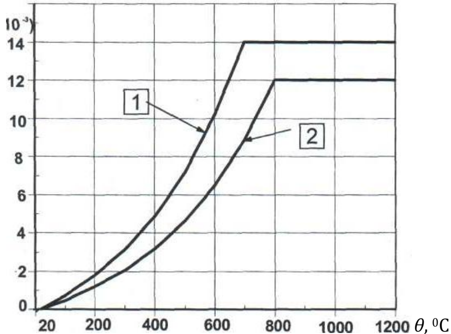
Рисунок 11.3 – Повне температурне розширення бетону:
