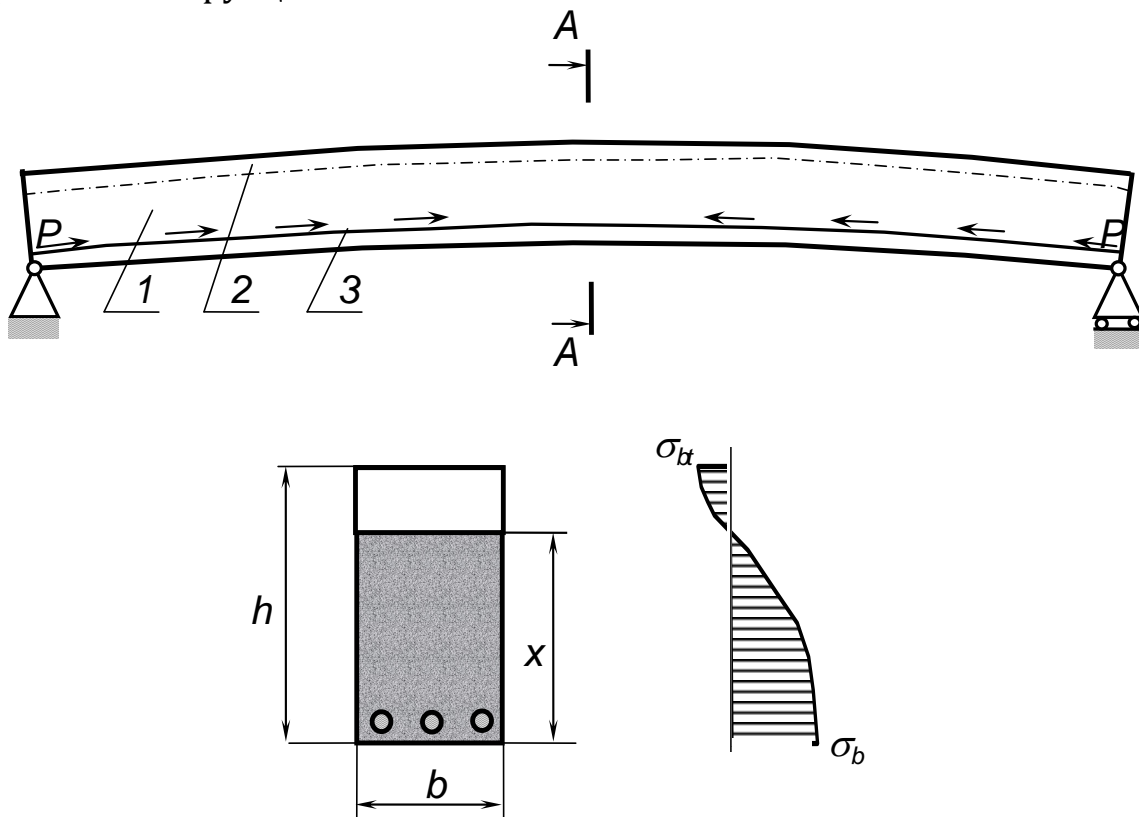
Рисунок 7.7 – Схема попередньо напруженої залізобетонної балки:
