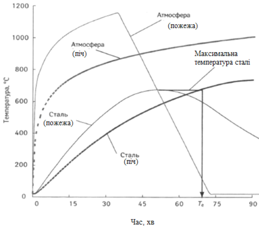
Рисунок 6.2 – Концепція еквівалентної тривалості пожежі на прикладі сталюого елемента конструкції, представлена доктором Б.Кірбі (B.Kirby)
