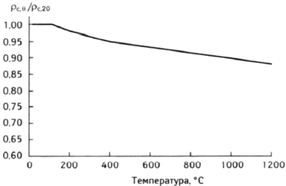
Рисунок 11.6 – Густина бетону за підвищених температур
