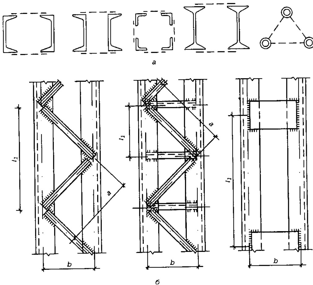
Рисунок 10.4 – Найпоширеніші види стержнів наскрізних колон:
