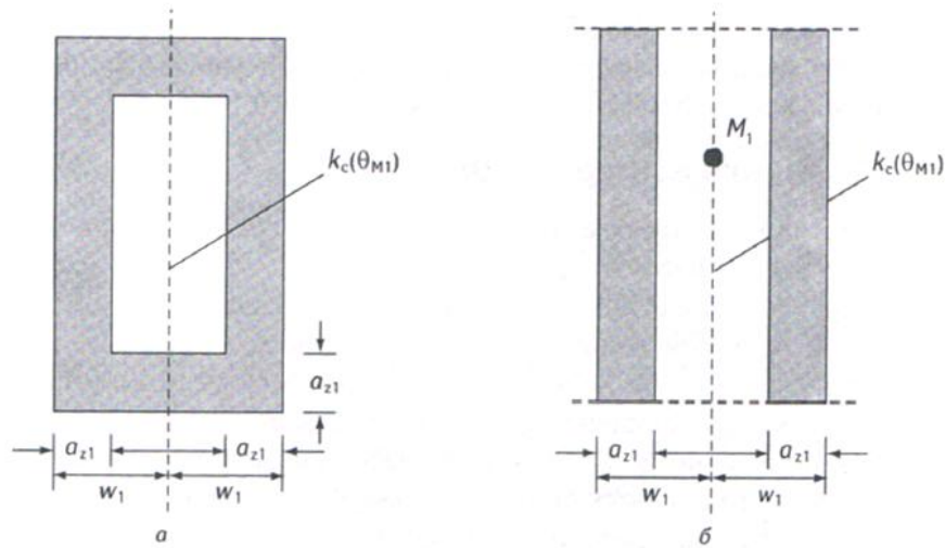
Рисунок 12.4 – Визначення зменшеного поперечного перерізу бетону для залізобетонних плит:
