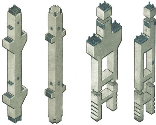
Рисунок 2.9 – Залізобетонні колони
