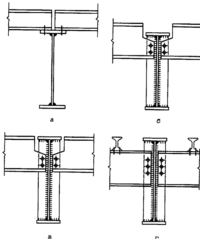
Рисунок 9.4 – Типи з'єднань балок: обпирання зверху:
