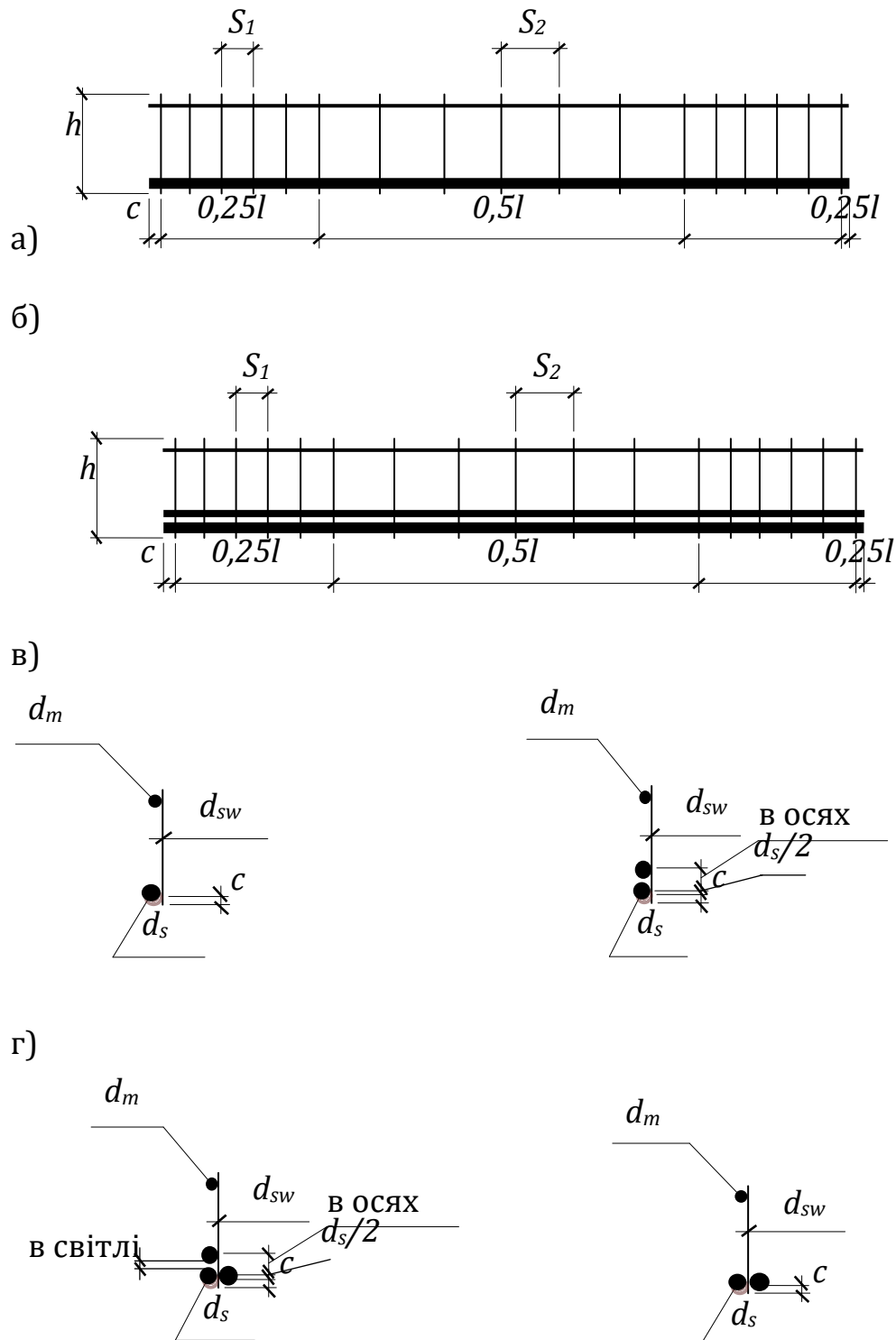
Рисунок 8.6 – Плоскі каркаси:
