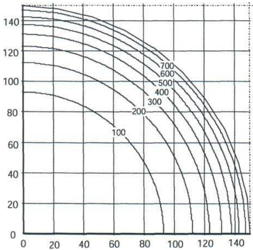
Рисунок 6.19 – Температурні криві круглої колони діаметром 300 мм – R30, °C
