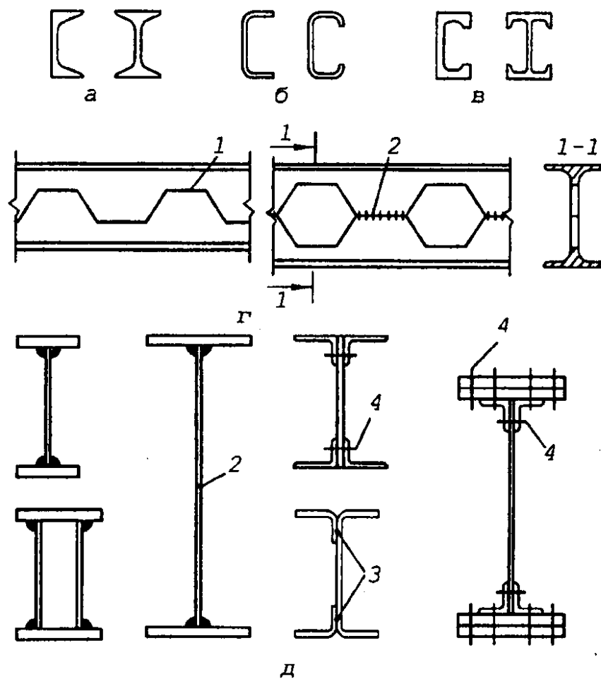
Рисунок 9.2 – Приклади найпоширеніших перерізів балок:
