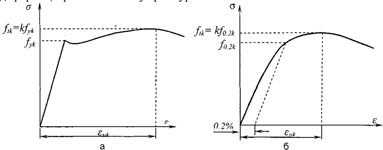
Рисунок 8.10 – Діаграма напруження-деформації розтягу для звичайної арматурної сталі :
