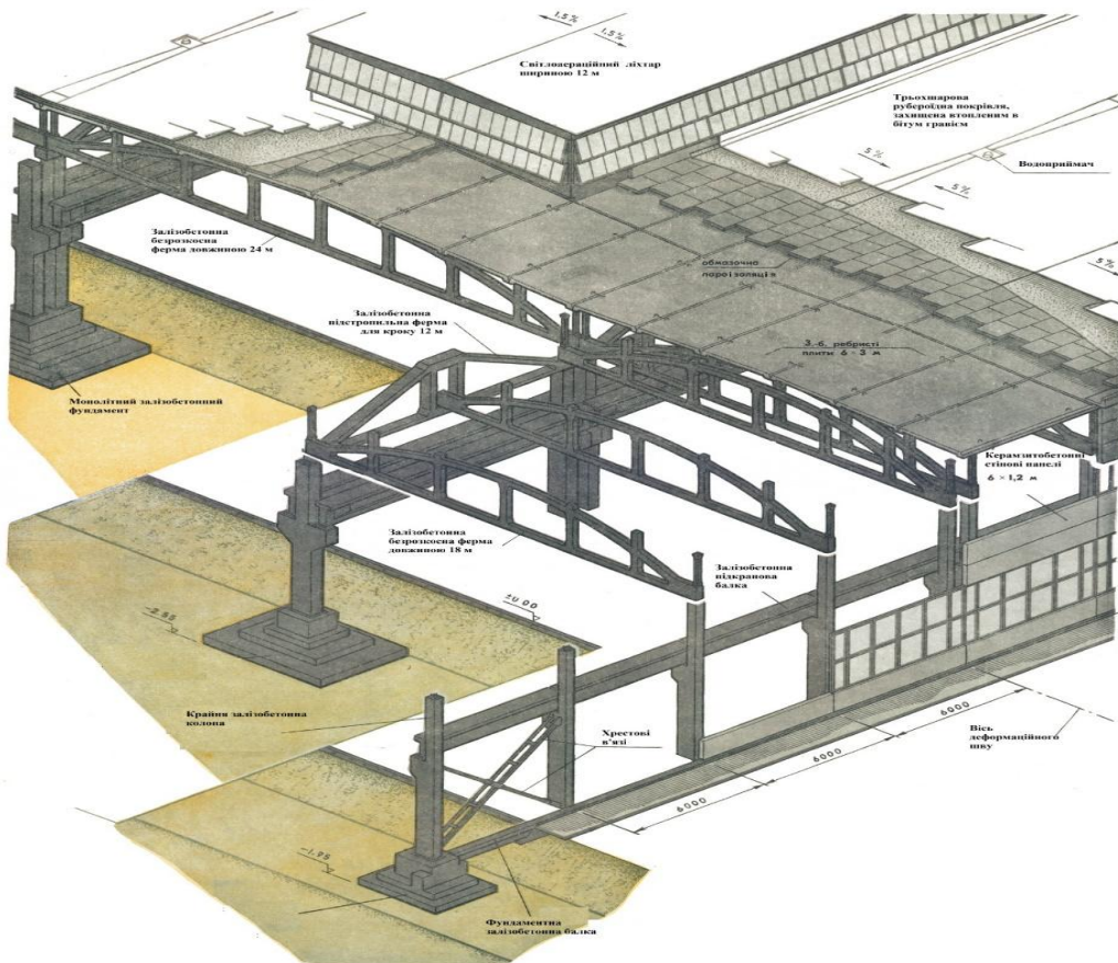
Рисунок 2.16 – Каркас промислової будівлі
