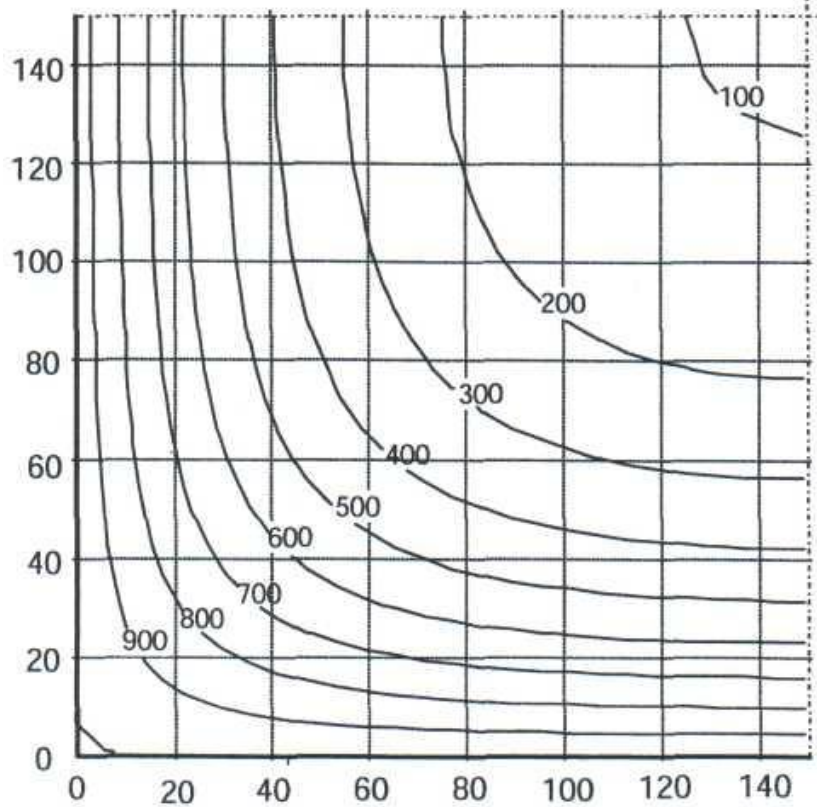
Рисунок 6.16 – Температурні криві колони h \times b = 300 \text{ мм} \times 300 \text{ мм} – R90, °C
