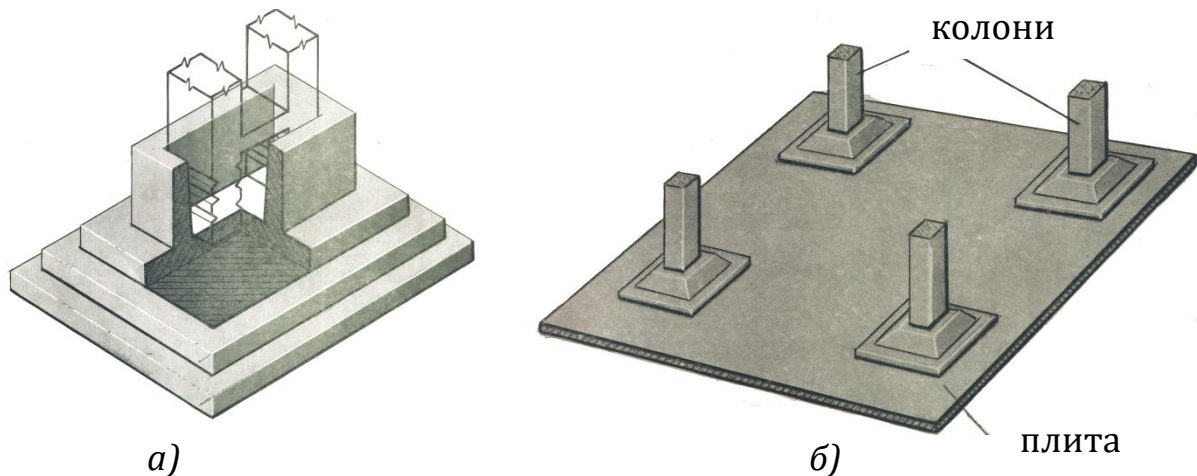
Рисунок 2.7 – Монолітний фундамент під колону (а) та монолітна плита під всю споруду (б)
