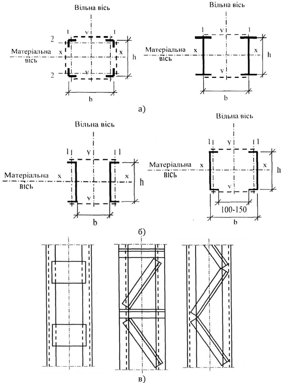
Рисунок 10.5 – Типи решіток наскрізних стержнів:
