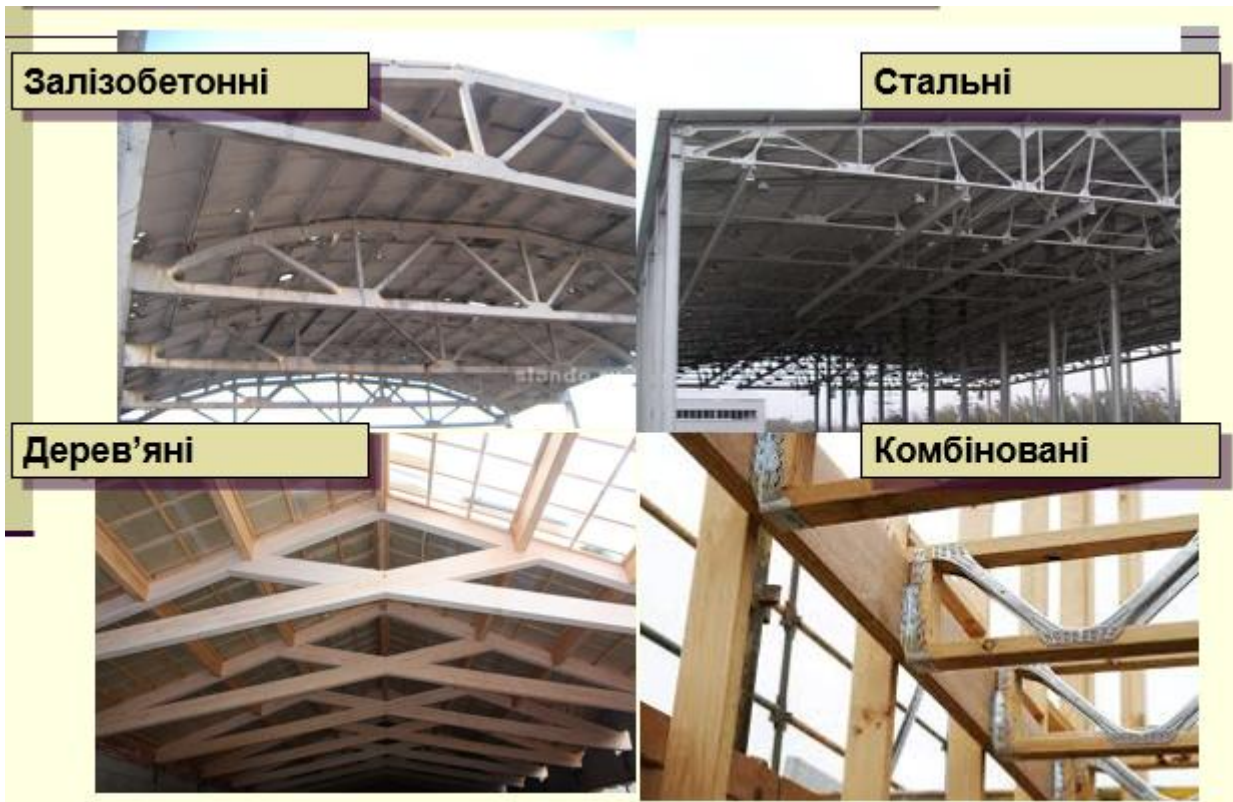
Рисунок 2.14 – Ферми покриття
