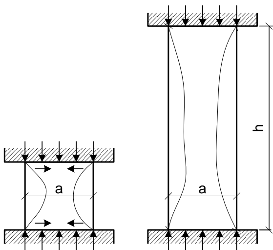
Рисунок 7.2 – Випробування бетонного куба та бетонної призми на стиск
