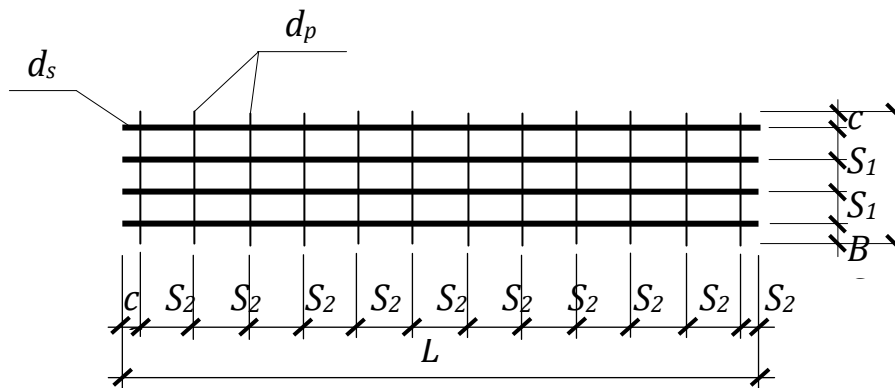
Рисунок 8.3 – Сітка з поздовжньою робочою арматурою
