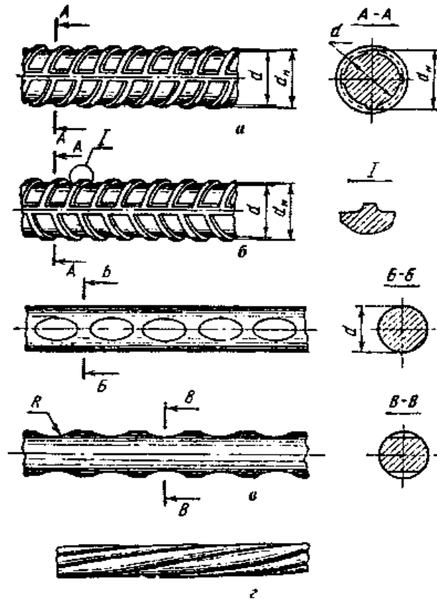
Рисунок 8.2 – Арматура:
