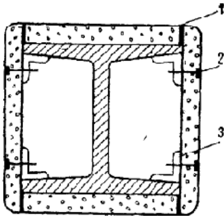
Рисунок 14.3 – Захист металевої колони збірними залізобетонними плитами:
