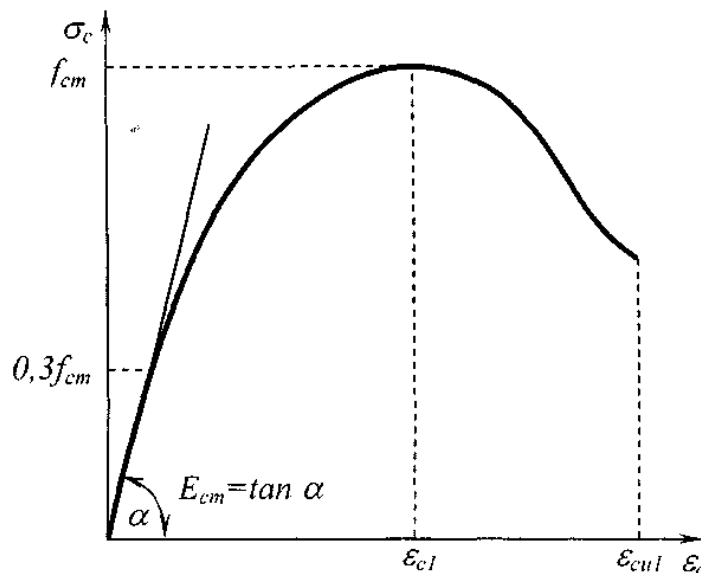
Рисунок 7.4 – Діаграма напруження-деформації бетону
