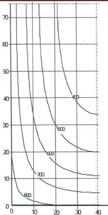
Рисунок 6.6 – Температурні криві балки h \times b = 150 \text{ мм} \times 80 \text{ мм} – R30, °C
