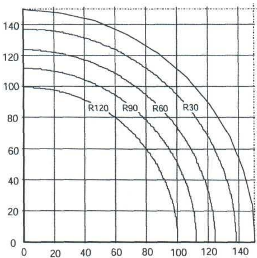
Рисунок 6.23 – Ізотерма 500 °C круглої колони діаметром 300 мм
