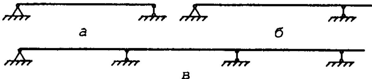
Рисунок 9.1 – Найпоширеніші статичні схеми балок:
