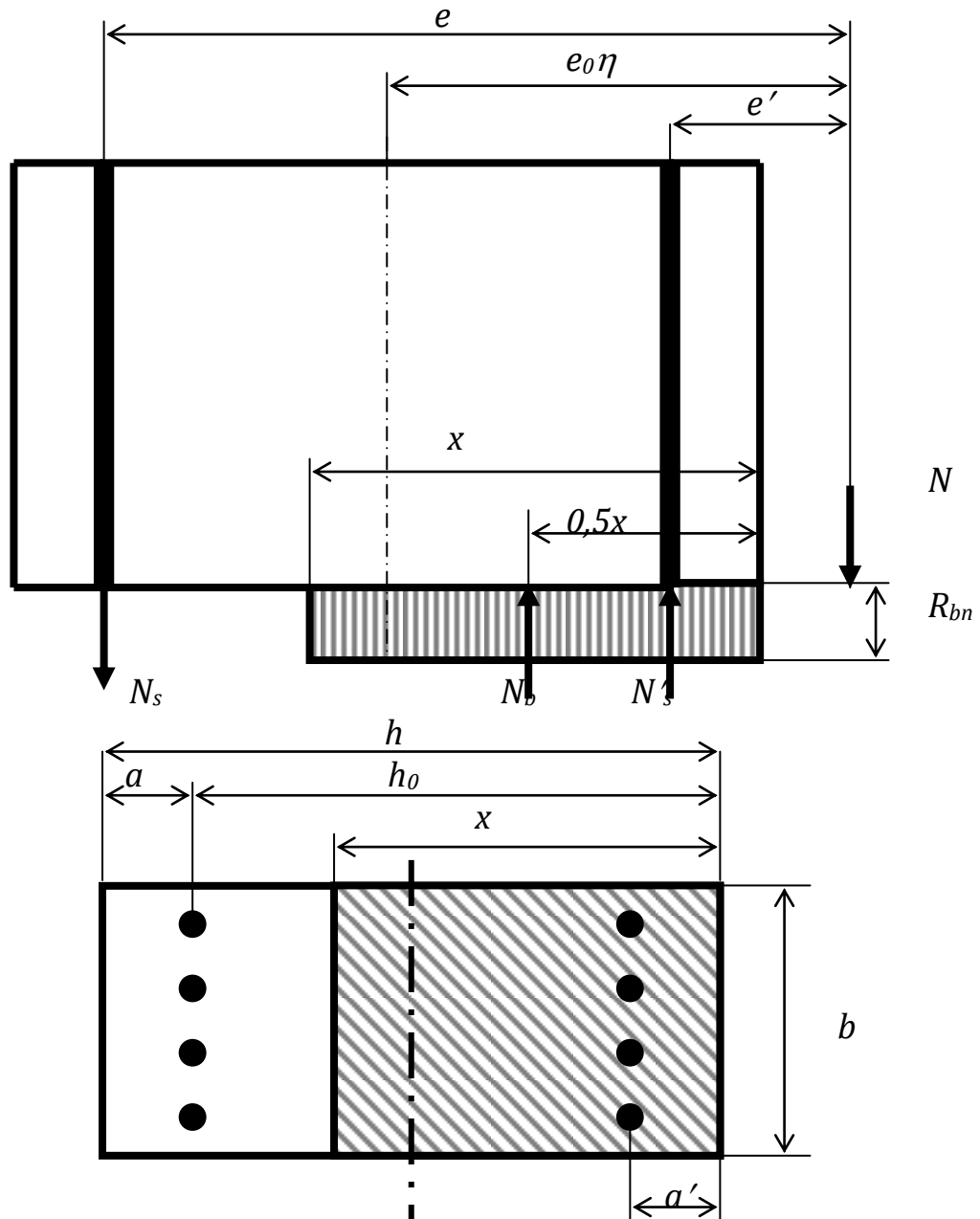
Рисунок 13.3 – Розрахункова схема залізобетонної колони для випадку 1, де: x – висота стиснутої зони бетону; R_{bn} – характеристичний опір бетону; b – ширина перерізу колони; R_{sn} – характеристичний опір арматури стиску і розтягу; A'_s, A_s – площа стиснутої і розтягнутої арматури відповідно
