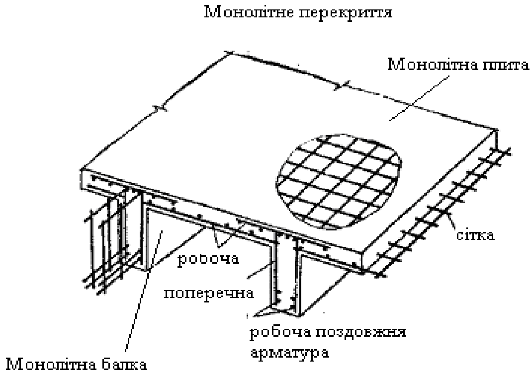
Рисунок 8.9 – Застосування арматури в монолітному перекритті
