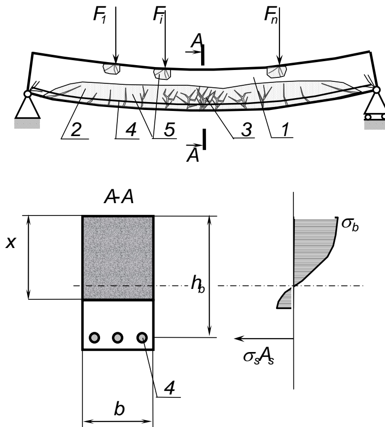
Рисунок 7.6 – Схема роботи залізобетонної балки на згин:
