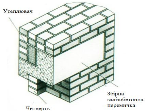
Рисунок 2.13 – Перемичка
