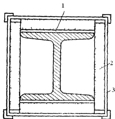
Рисунок 14.5 – Захист вермикулітовими плитами:
