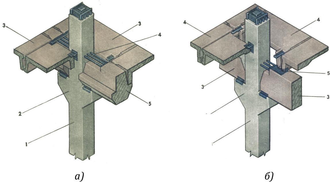
Рисунок 2.10 – З'єднання залізобетонних колон з конструкціями перекриття:
