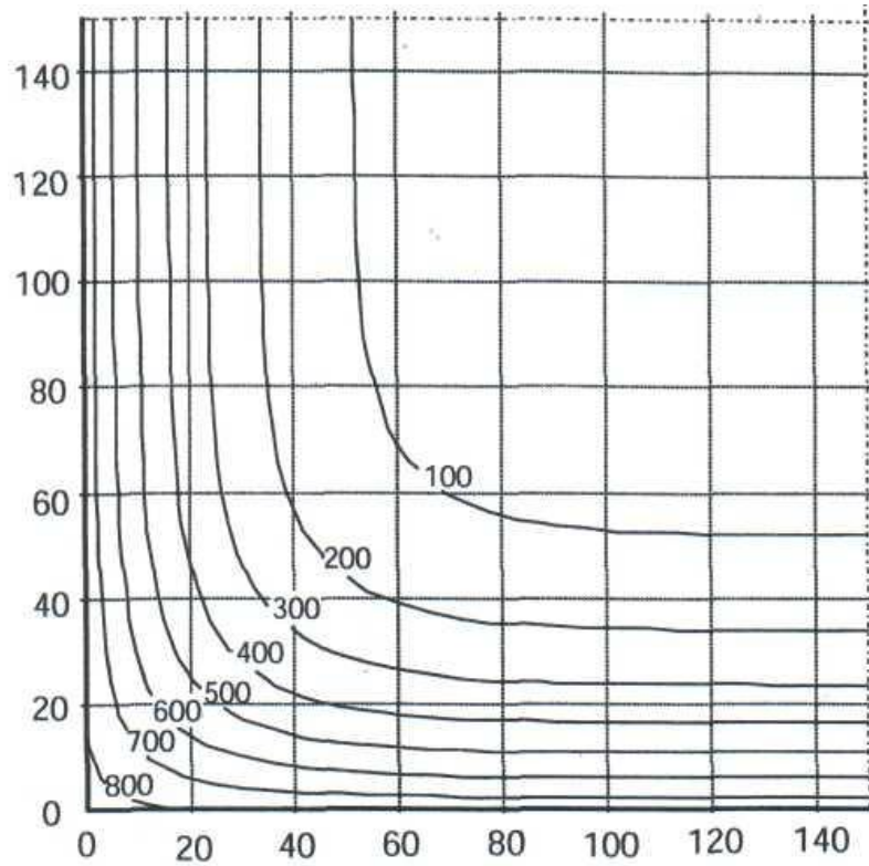
Рисунок 6.14 – Температурні криві колони h \times b = 300 \text{ мм} \times 300 \text{ мм} - R30, ^\circ\text{C}
