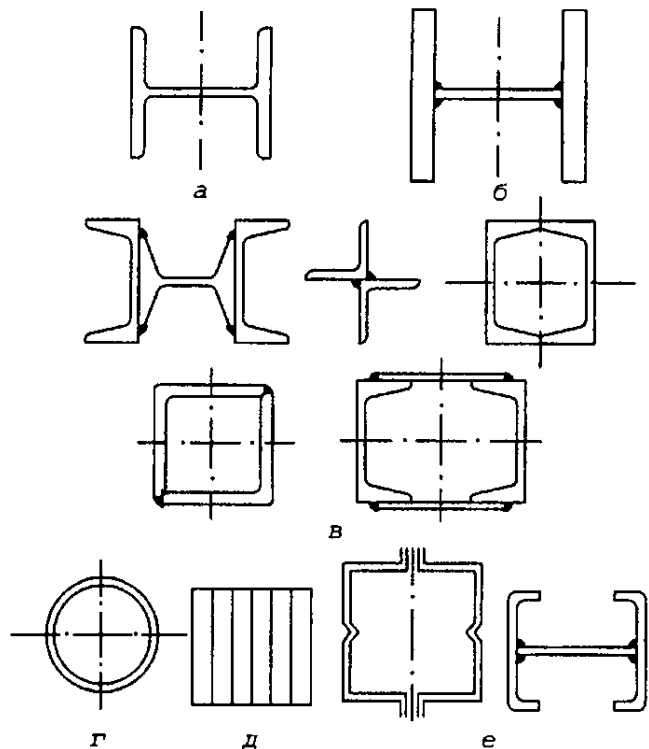
Рисунок 10.3 – Поширені типи перерізів суцільних колон
