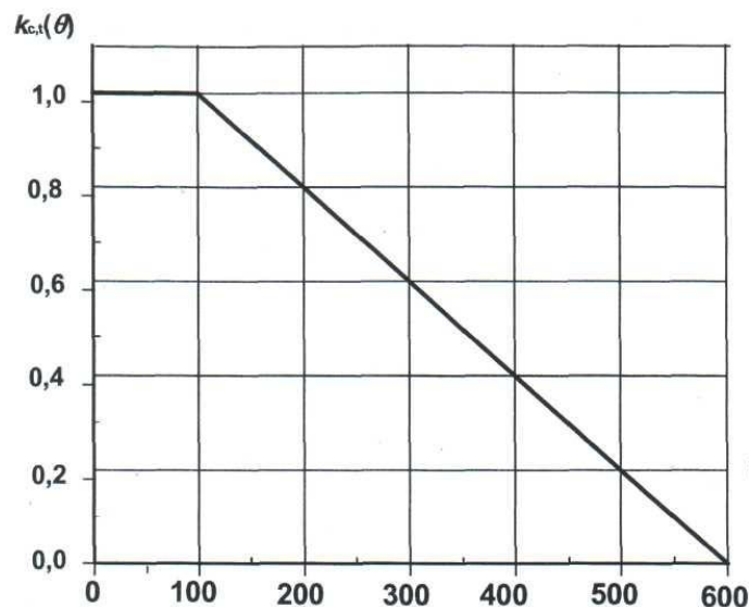
Рисунок 11.2 – Коефіцієнт k_{c,t}(\theta) зниження опору бетону на розтяг ( f_{ck,t} ) за підвищених температур
