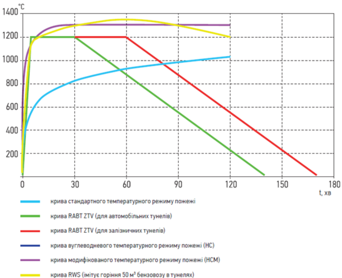
Рисунок 6.1 – Номінальні режими пожежі: порівняння з результатами випробувань вогнестійкості при реальній пожежі
