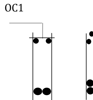
Рисунок 8.8 – Здвоєні каркаси
