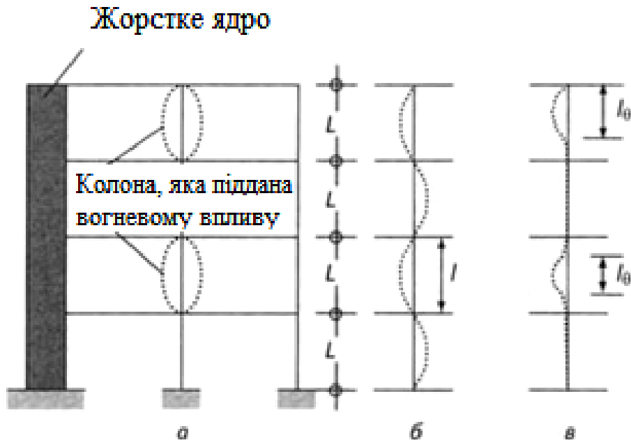
Рисунок 13.5 – Розрахункова довжина колони у жорсткому каркасі при впливі пожежі:
