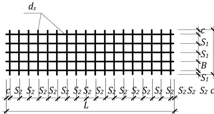
Рисунок 8.5 – Сітка з робочою арматурою в двох напрямках
