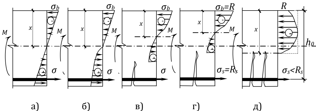
Рисунок 12.1- Стадії напружено-деформованого стану при згині:
