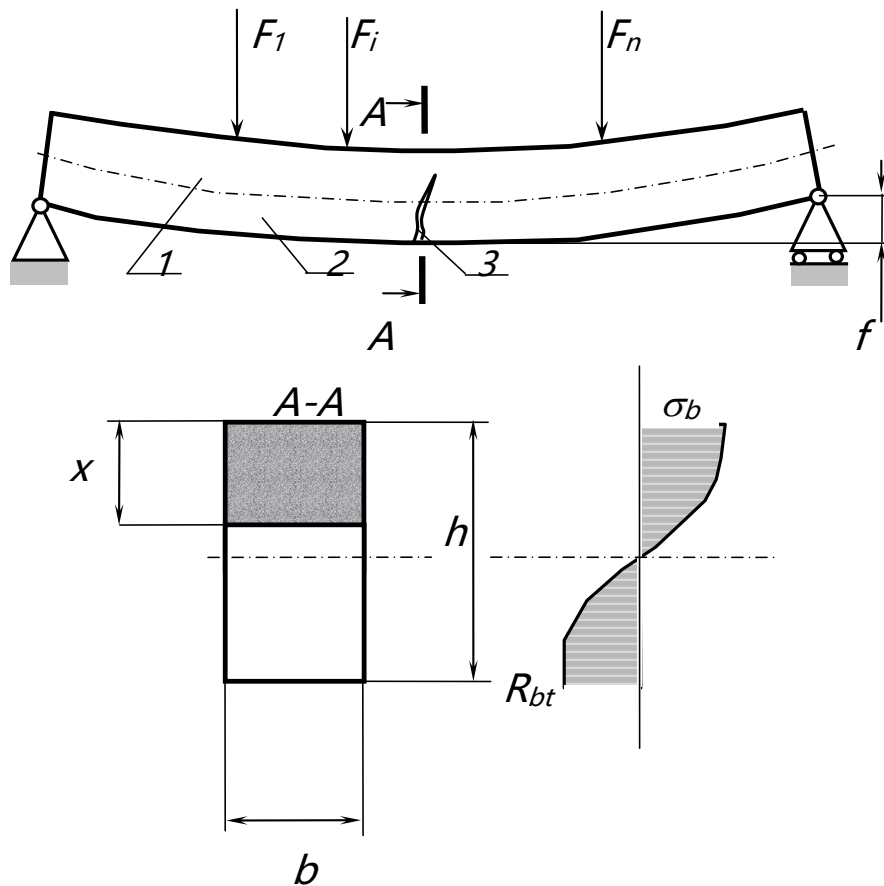
Рисунок 7.5 – Схема роботи бетонної балки на згин:
