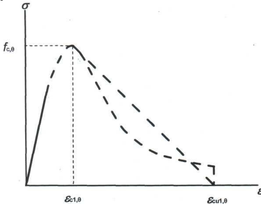
Рисунок 11.1 – Математична модель діаграми «напруження-деформація» стиснутого бетону за підвищених температур
