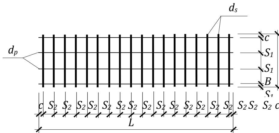
Рисунок 8.4 – Сітка з поперечною робочою арматурою
