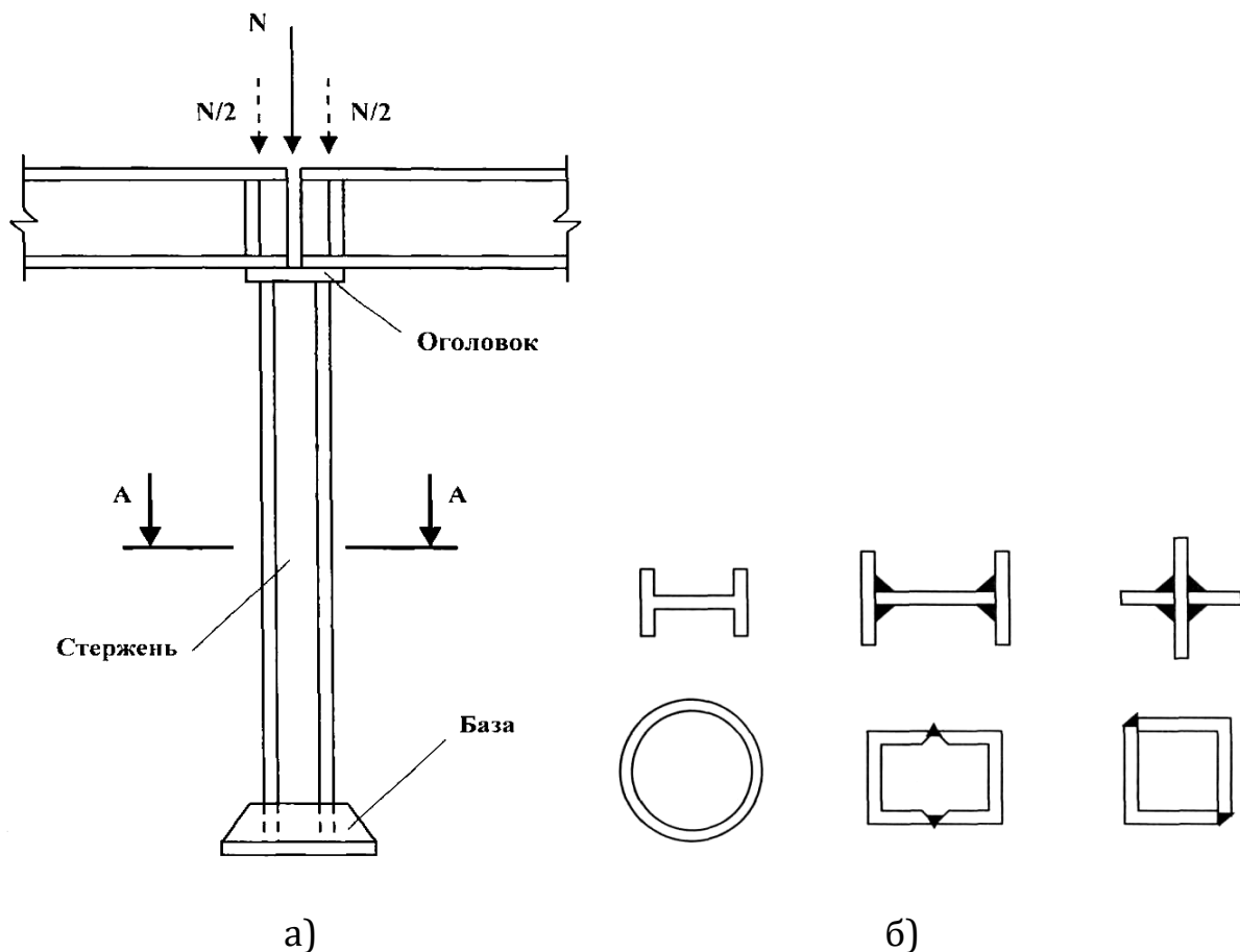
Рисунок 10.1 – Суцільні колони :
