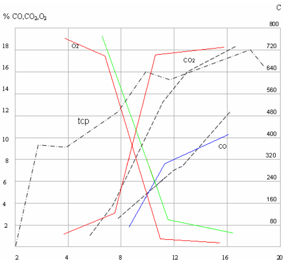
Рис. 2. Зміна вмісту продуктів горіння в купе: tcp- середньоб'ємна температура.
