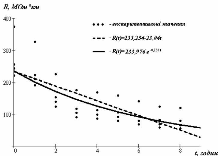
Рис. 3 – Показова та лінійна моделі залежності опору ізоляції від часу експлуатації з накладанням на експериментальні точки для кабелю марки АВВГ 4x10
