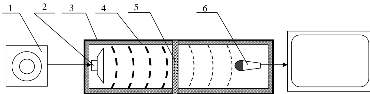
Рис.1 Схема установки
