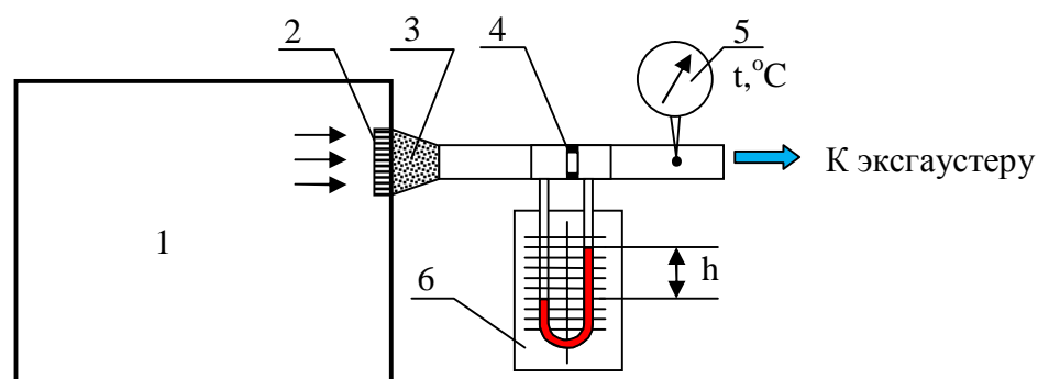
Рис.1 Схема установки
