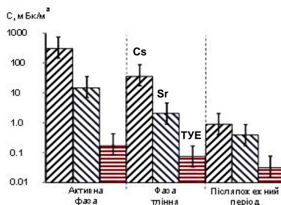
Рис. 2 – Об'ємна активність радіонуклідів у атмосферному повітрі при різних фазах лісової пожежі
