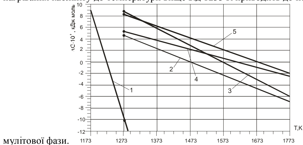
Рис. 1. Залежність енергії Гіббса ( \Delta G ) від температури (Т) при нагріванні: 1 - каоліну; 2 - AL_2O_3 - SiO_2 ам.; 3 - AL_2O_3 - SiO_2 кр.; 4 - ZrO_2 \cdot SiO_2 ам.; 5 - ZrO_2 \cdot SiO_2 кр.
