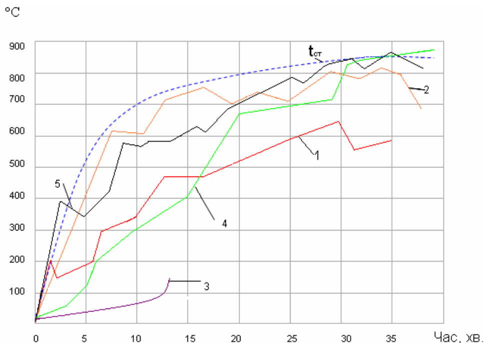
Рис. 1. Температурний режим при горінні в макетах; t_{ст} - температурна крива стандартної пожежі; 1, 2 - середньооб'ємна температура в купе (у першому досліді). 4, 5 - середньооб'ємна температура в купе (у другому досліді). 3 - температура за вогнезатримуючою перегородкою.
