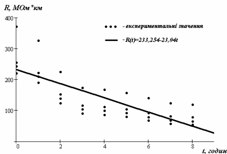
Рис. 1 – Лінійна модель залежності опору ізоляції від часу експлуатації з накладанням на експериментальні точки для кабелю марки АВВГ 4х10
