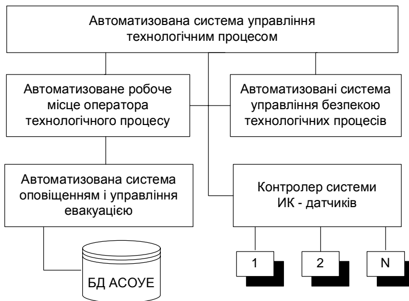
Рис. 1. Розподіл інформаційних потоків у системі АСУТП - АСУБТП - АСОУЕ
