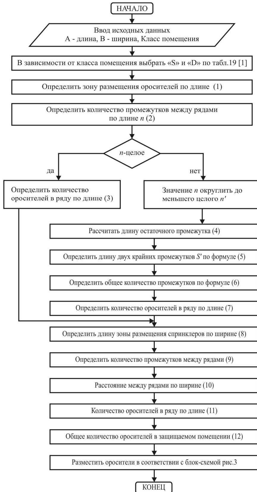
Рисунок 1 – Блок-схема алгоритма размещения оросителей
