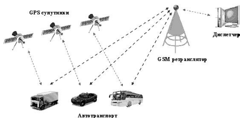
Рис. 1 - Принцип роботи системи GPS моніторингу
