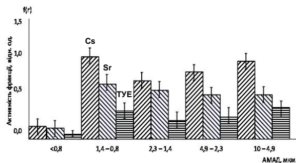
Рис. 6 – Розподіл активності радіонуклідів за розмірами по АМАД в РПЗ в активній фазі лісової пожежі
