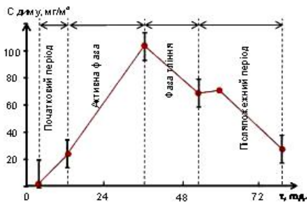
Рис. 1 – Показник вмісту концентрації диму в повітрі у місці лісової пожежі
