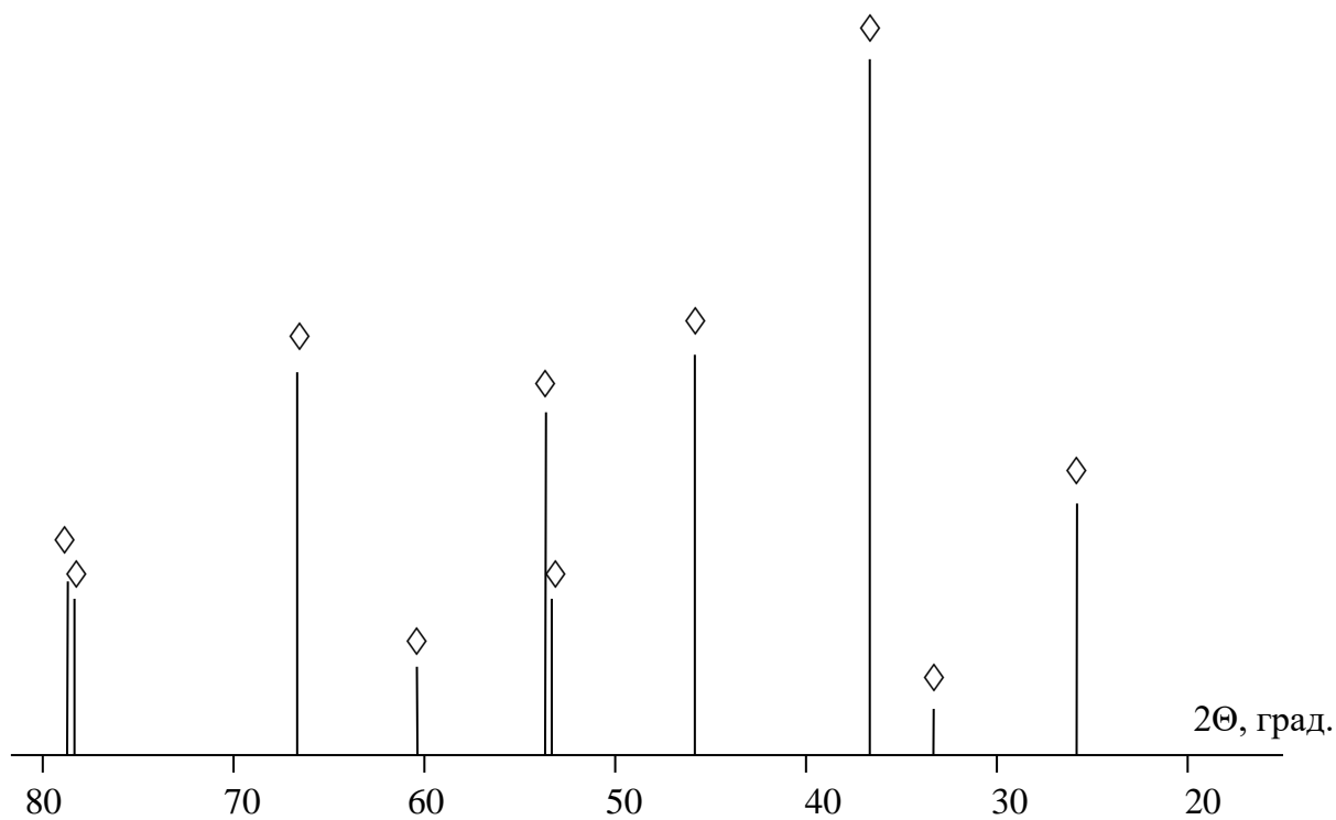
Рис. 3. Штрих-рентгенограмма синтезированного сегнетокерамического материала
