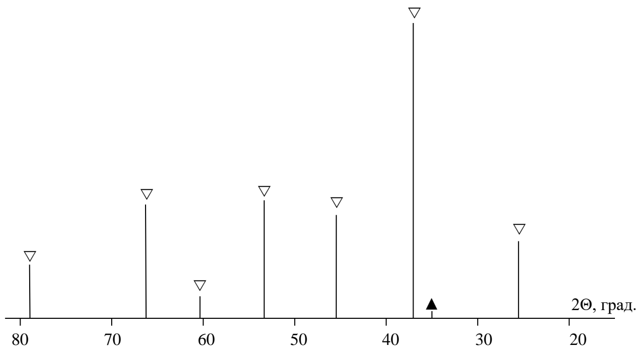
Рис. 4. Штрих-рентгенограмма сегнетокерамического материала образца :
