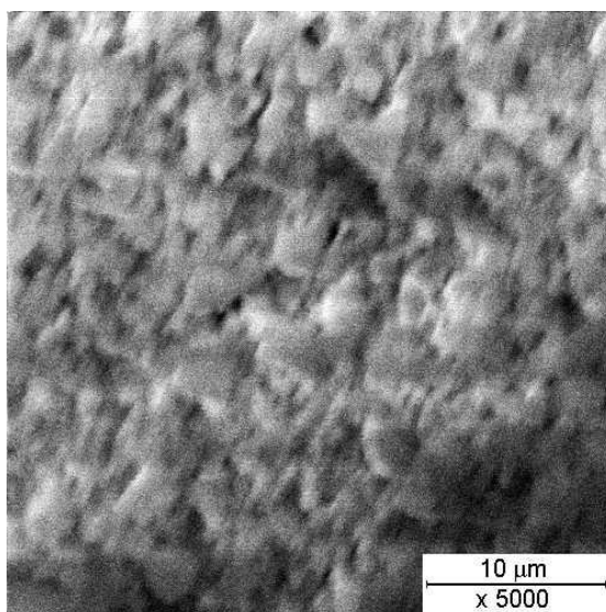
Рис. 5. Электронная фотография поверхности сегнетокерамического материала оптимального состава
