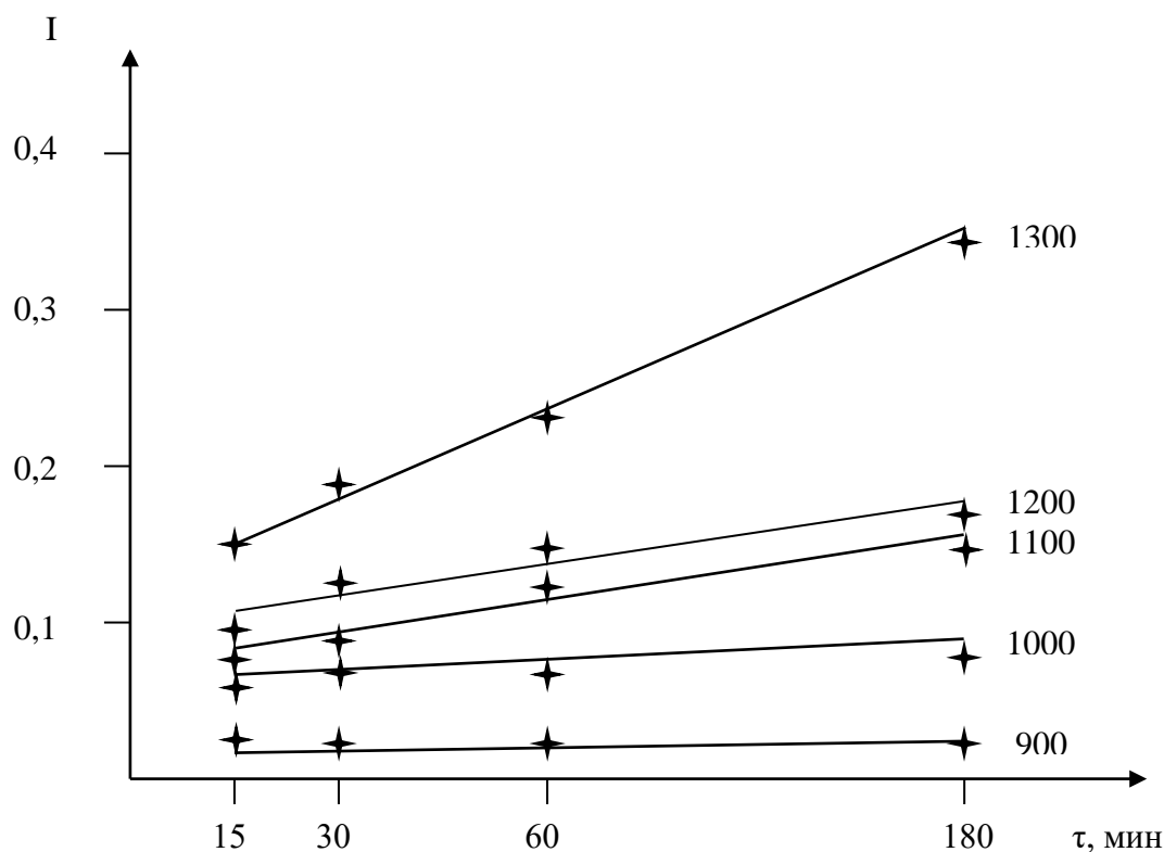
Рис. 2. Зависимость скорости реакции от температуры и времени выдержки
