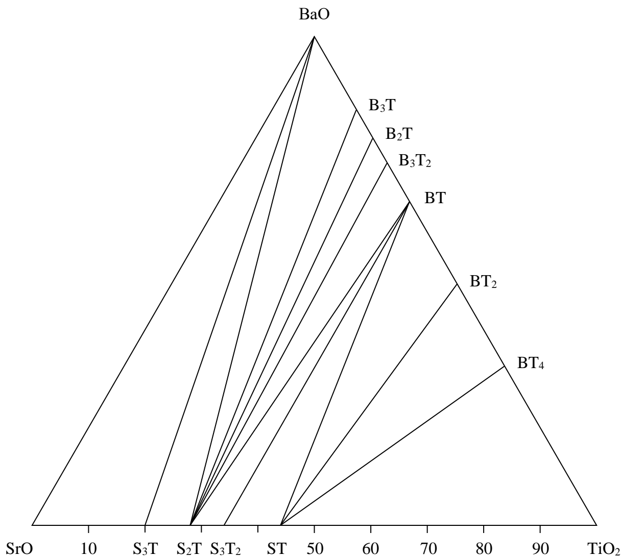
Рис. 1. Триангуляция системы \text{BaO} - \text{SrO} - \text{TiO}_2 при 1380\text{ }^\circ\text{C}
