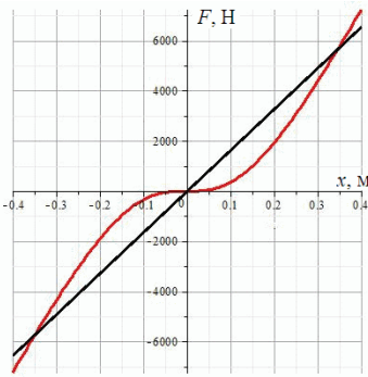
Рисунок 3 – Нелінійна пружна сила
