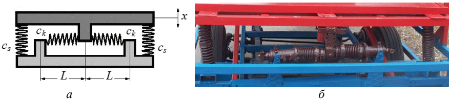
Рисунок 2 – Схема конструкції (а) та фотографія дослідного зразку (б) другої ступені ресорного підвішування, що реалізує квазінульову жорсткість
