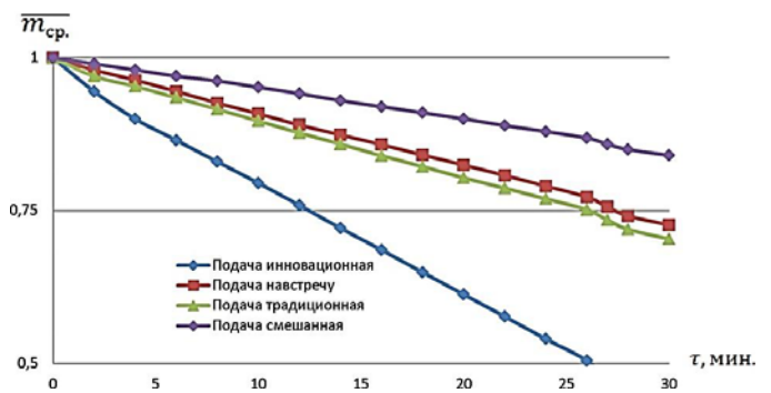
Рис. 3 – Дослідження втрати маси октану при різних схемах подачі припливного повітря
