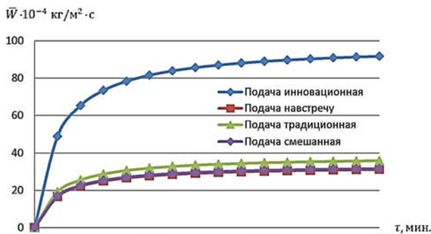
Рис. 17 – Графік середнього значення інтенсивності випару толуолу
