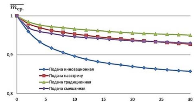
Рис. 6 – Дослідження втрати маси дизельного палива при різних схемах подачі припливного повітря
