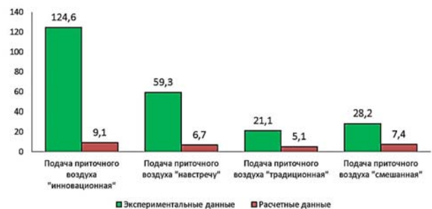
Рис. 13 – Діаграма втрати маси толуолу при вентиляції резервуара
