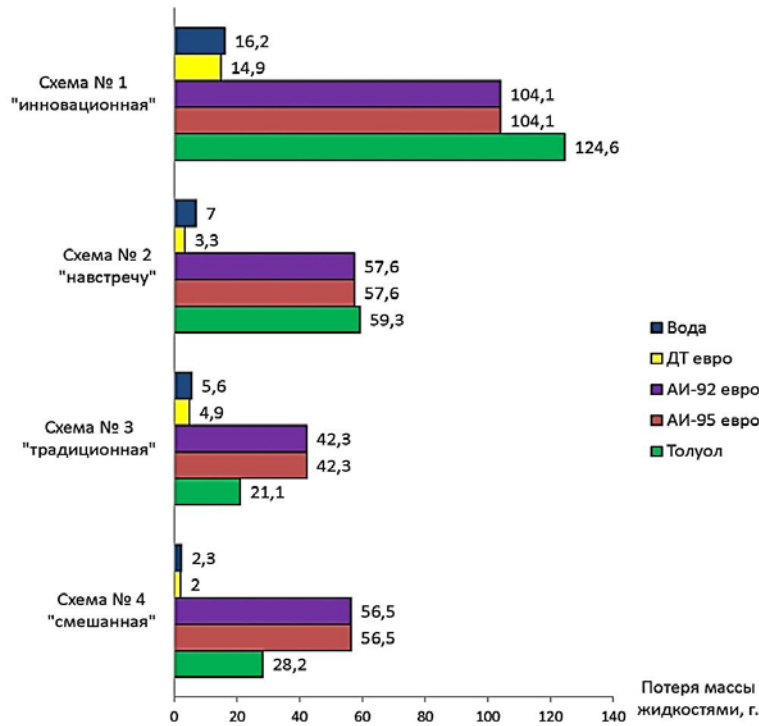
Рис. 14 – Залежність втрати маси рідин за 1 годину вентиляції, отримана експериментальним шляхом
