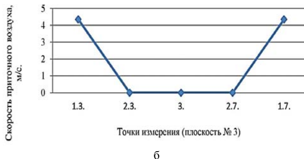
Рис. 8 – Графіки зміни інтенсивності випару толуолу залежно від рухливості повітря над поверхнею випару в експериментальному резервуарі при подачі припливного повітря запропонованим способом: а – графік зміни втрати маси толуолу в площині перетину III; б – графік зміни швидкості припливного повітря в площині перетину III
