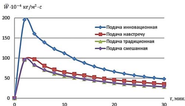
Рис. 18 – Графік середнього значення інтенсивності випару бензинів А-92/95
