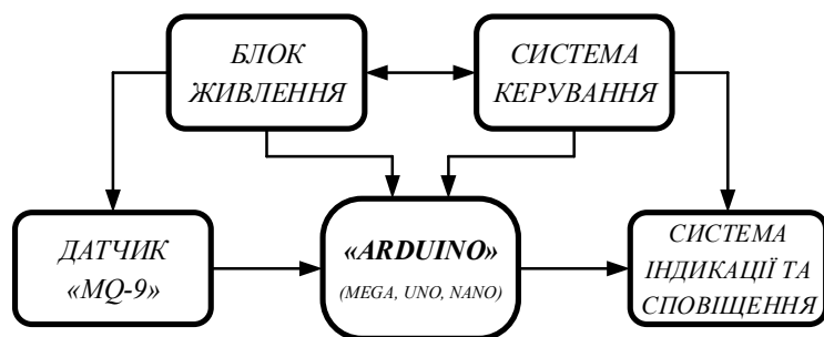
Рисунок 1 – Структурна схема газоаналізатора з датчиком «MQ-9»
