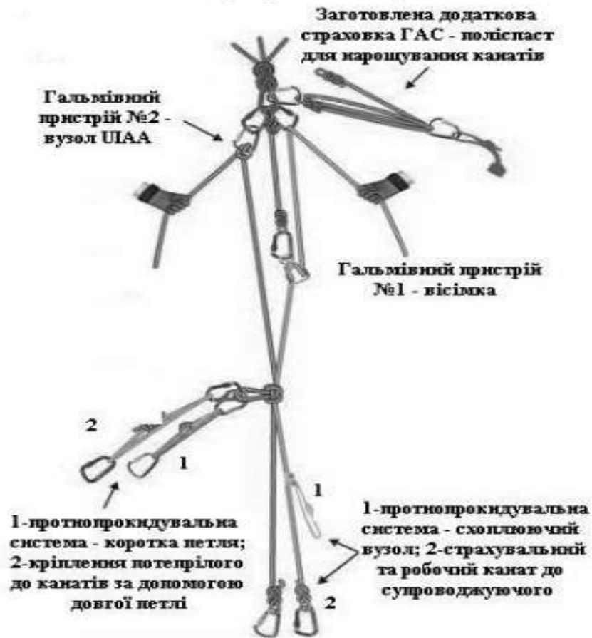
Рису. 1 – Кріплення потерпілого та супроводжувача до спускових канатів та приклади організації протипрокидувальних систем
