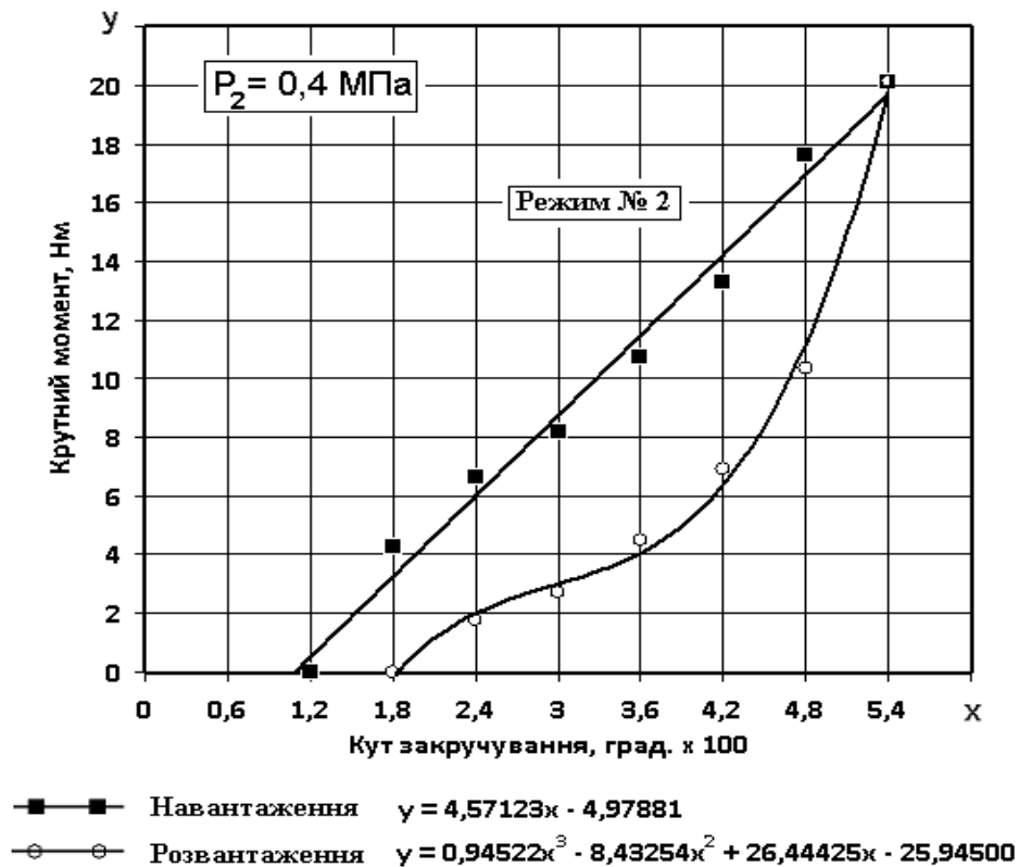
Рис. 7 – Графіки режиму навантаження – розвантаження № 2
