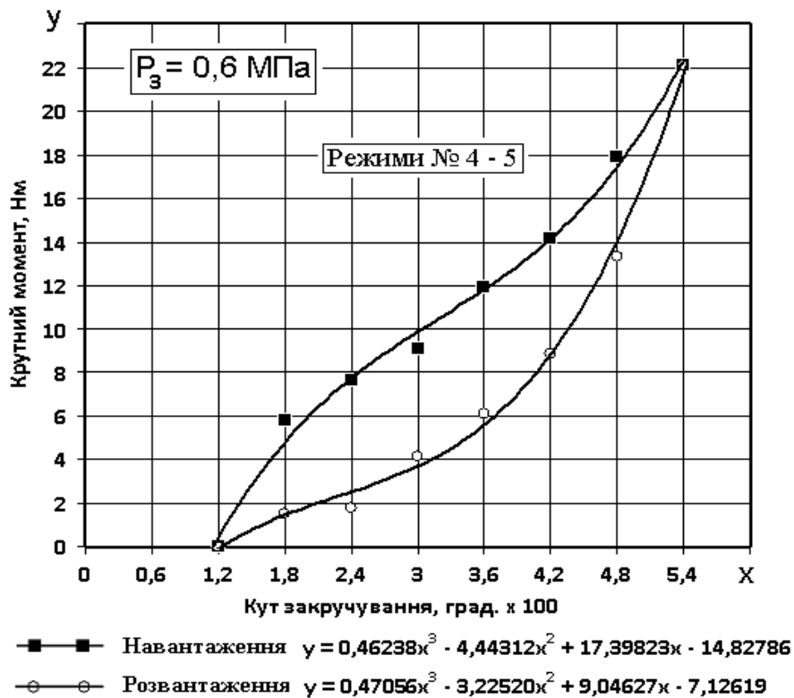
Рис. 13 – Графіки режимів навантаження - розвантаження № 4-5
