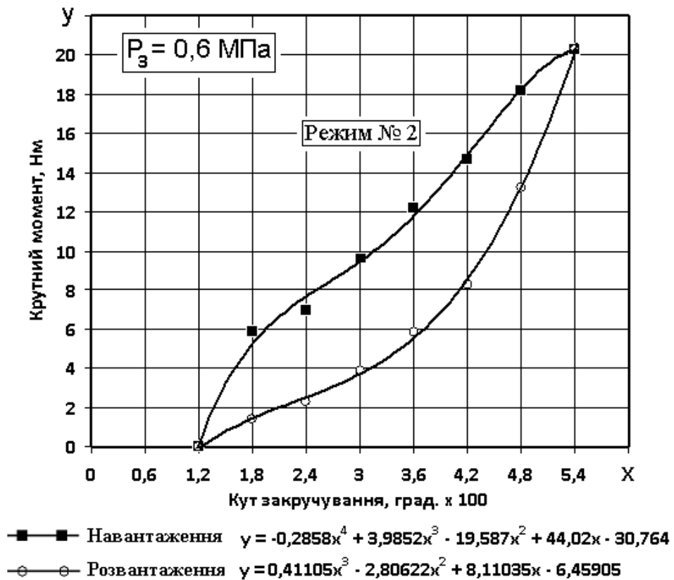
Рис. 11 – Графіки режиму навантаження – розвантаження № 2
