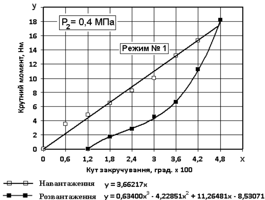
Рис. 6 – Графіки режиму навантаження – розвантаження № 1
