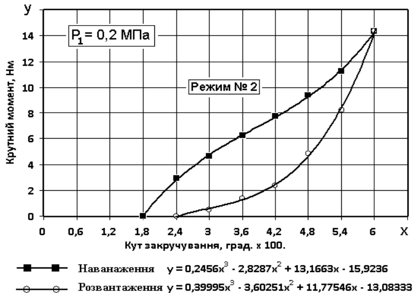
Рис. 3 – Графіки режиму навантаження – розвантаження № 2
