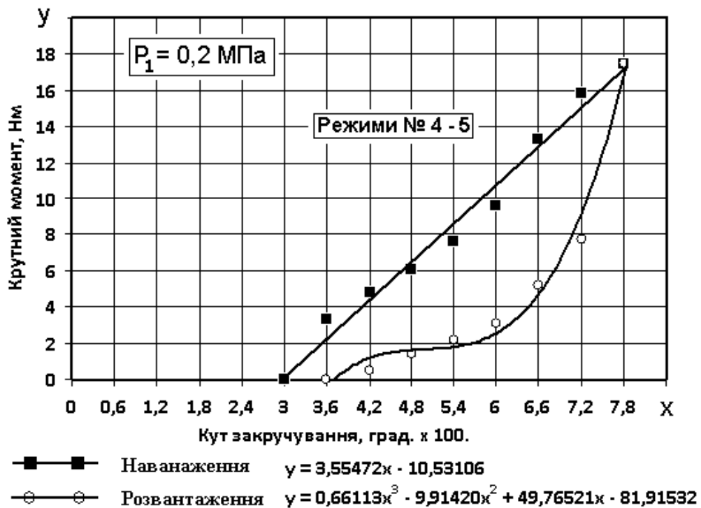
Рис. 5 – Графіки режимів навантаження - розвантаження № 4-5
