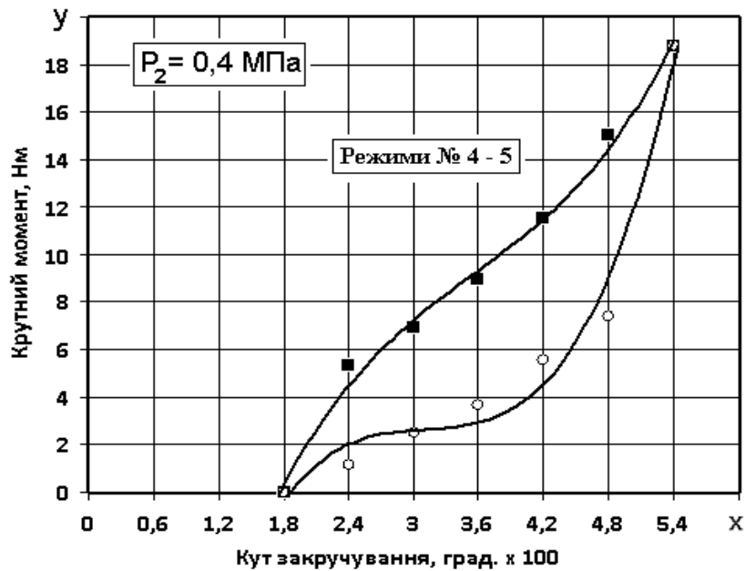
Рис. 8 – Графіки режиму навантаження – розвантаження № 3
