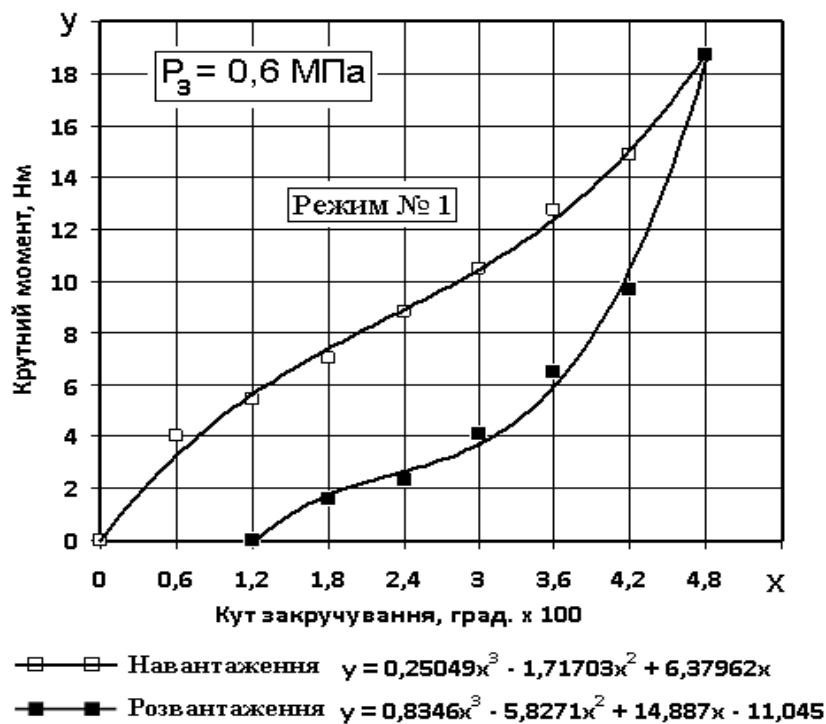
Рис. 10 – Графіки режиму навантаження – розвантаження № 1
