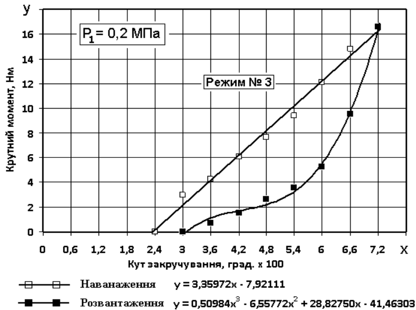
Рис. 4 – Графіки режиму навантаження – розвантаження № 3
