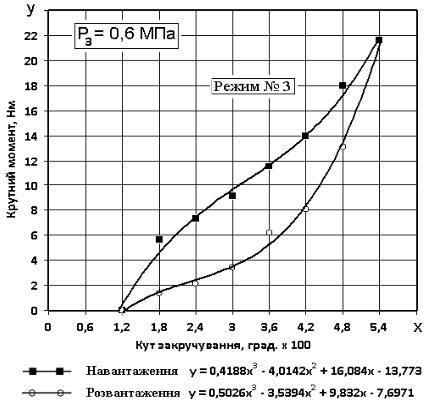
Рис. 12 – Графіки режиму навантаження – розвантаження № 3
